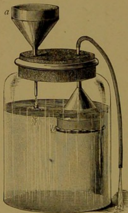
FIG. 3.—FILTERING-BOTTLE
