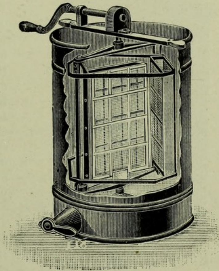
Fig. 60.—"Cowan" Rapid Extractor.
