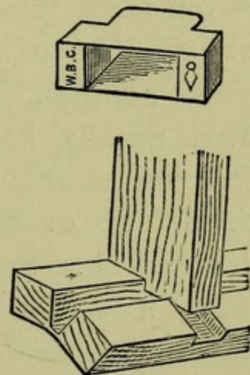
Fig. 44.—Meadows' Frame.
