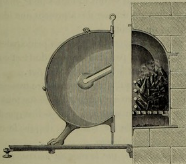
Fig. 17. Coupe du fourneau-modèle montrant l'appareil pour rôtir.
