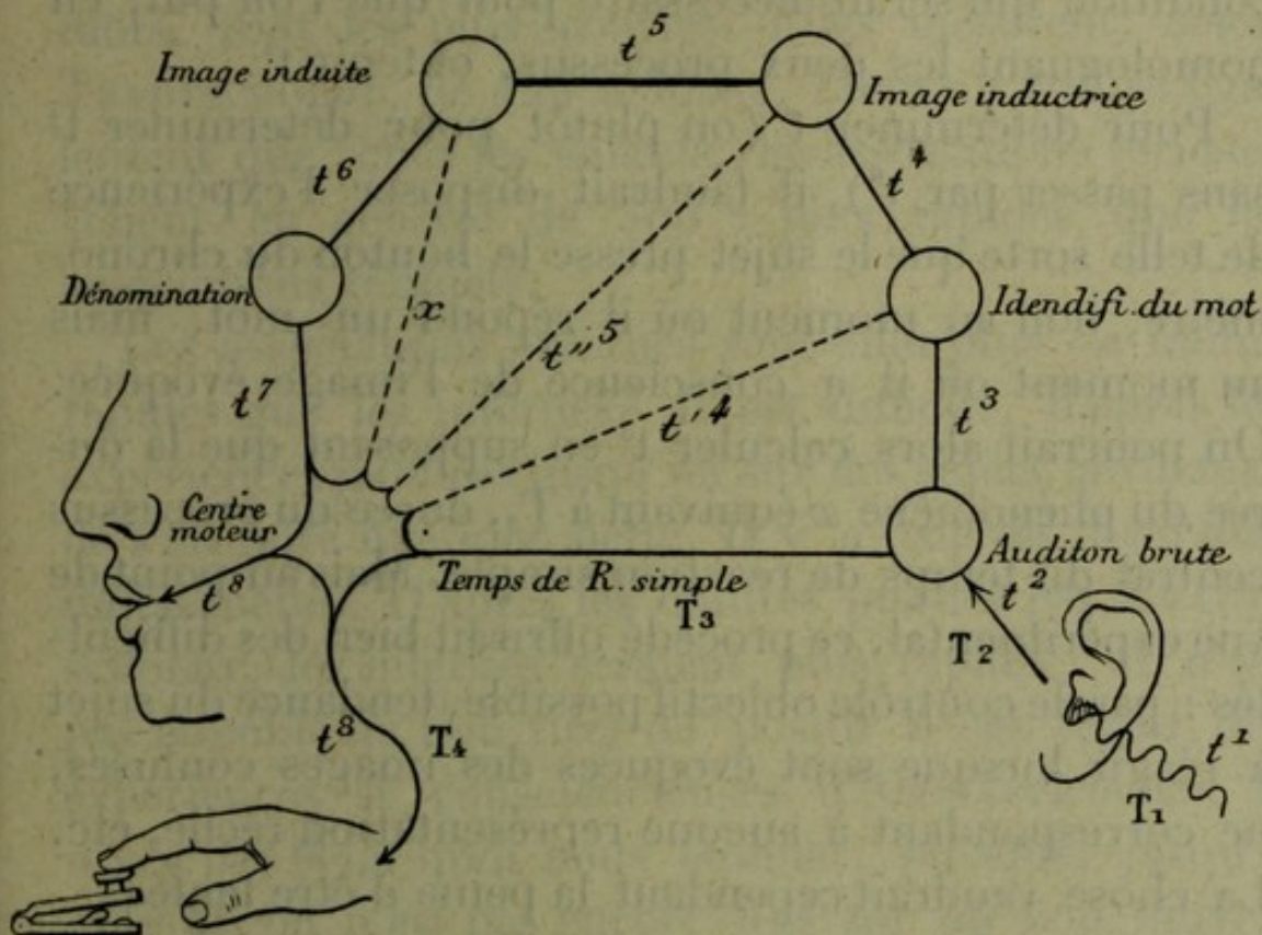
Fig. 6. — Temps d'association.
