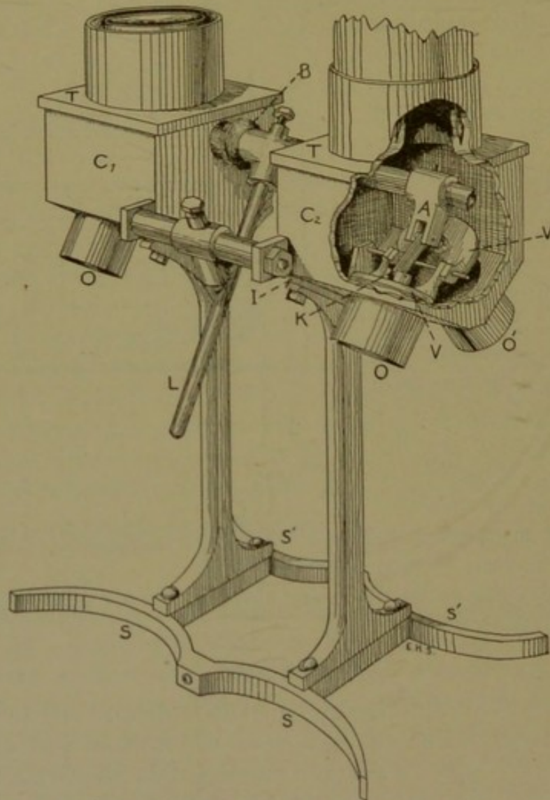
FIG. 3.—Valve box.
