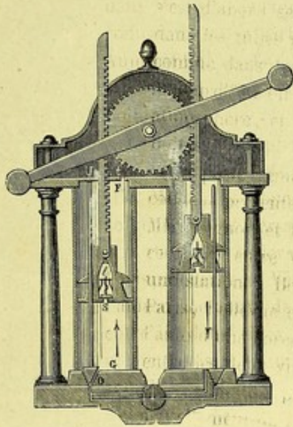
Corps de pompe et pistons de la machine pneumatique.
