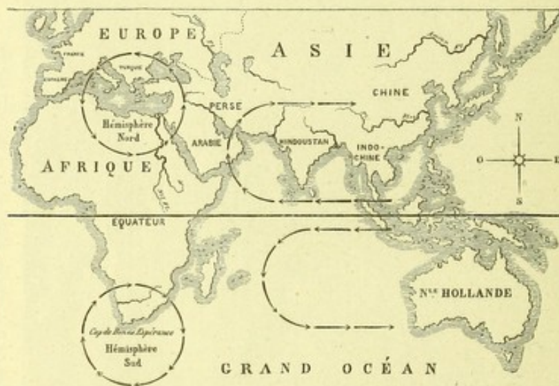
Mouvement de rotation et de translation des cyclones.
