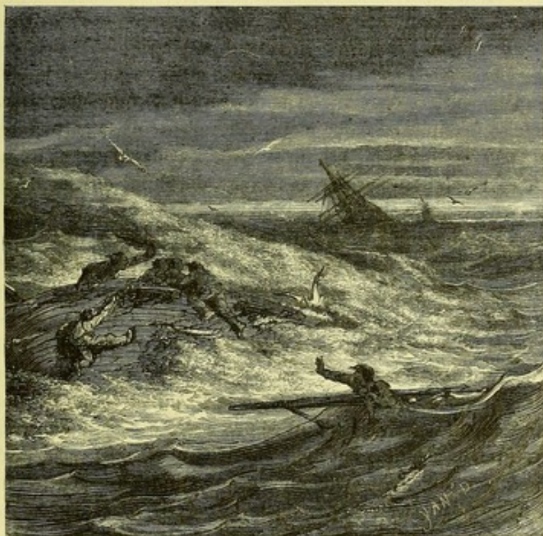
Cyclone sur la côte de Mozambique.
