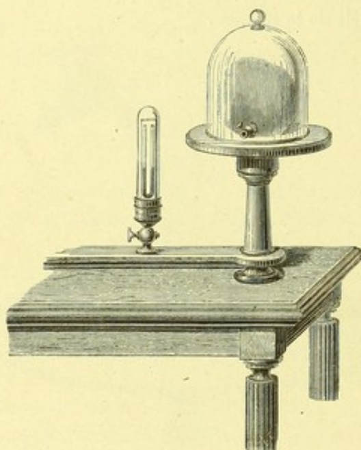
Dilatation des gaz dans le vide.
