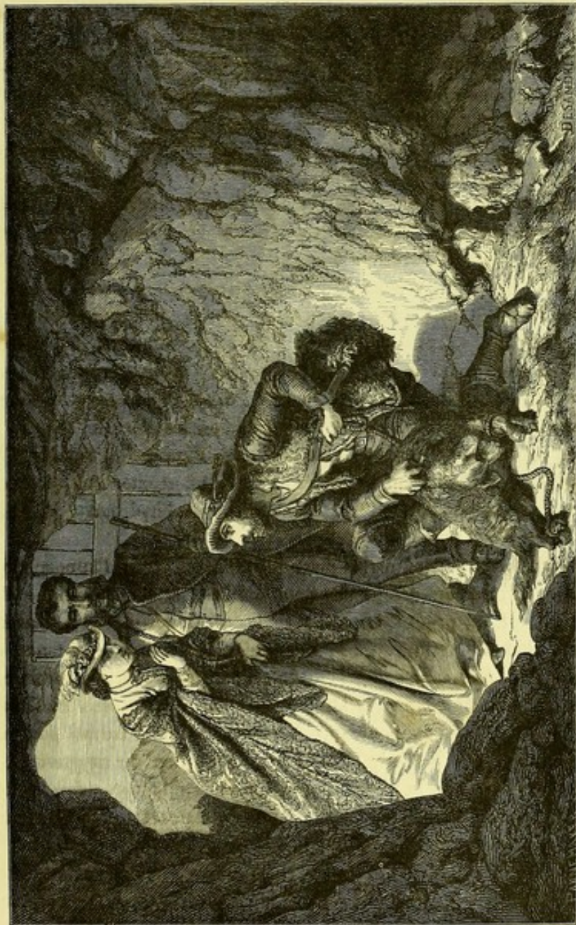
La grotte du Chien près de Pouzzoles.
