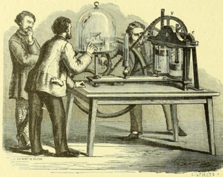
Machine pneumatique à deux cylindres.
