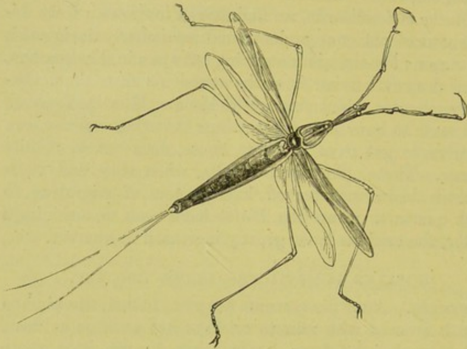
RANATRA LINEARIS.
