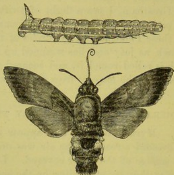
SPHINX STELLATARUM.
