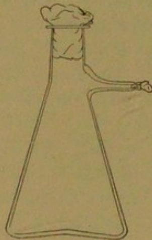
FIG. 7.—Filter flask.
