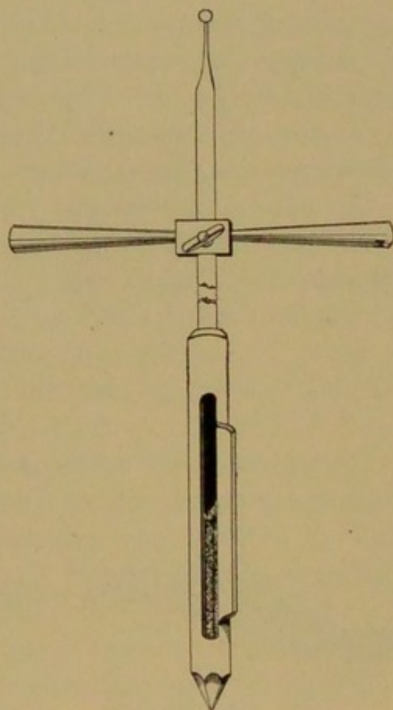
FIG. 218.—Fraenkel's borer.
