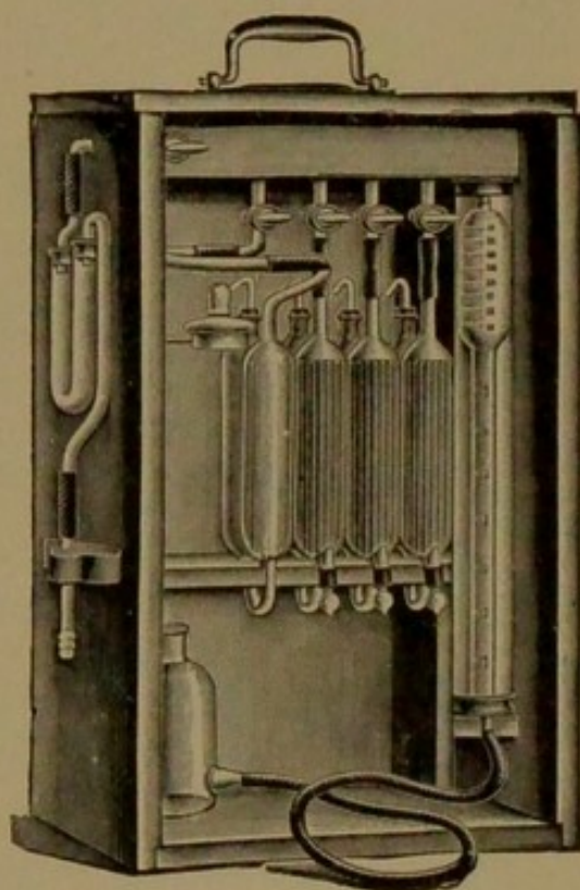
FIG. 154.—Orsat-Lunge gas analysis apparatus.
