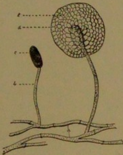
FIG. 77.— Mucor mucedo .
