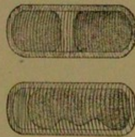
FIG. 86.—Plasmolysis.
