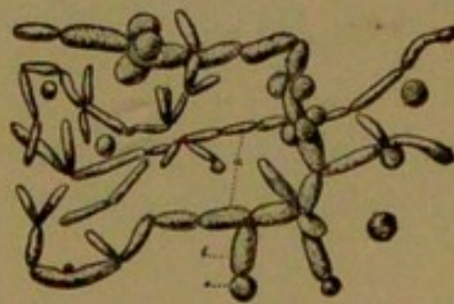
FIG. 82.— Torula .
