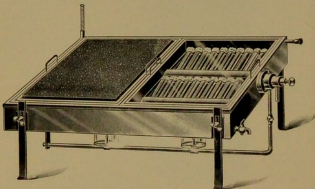
FIG. 110.—Serum inspissator.
