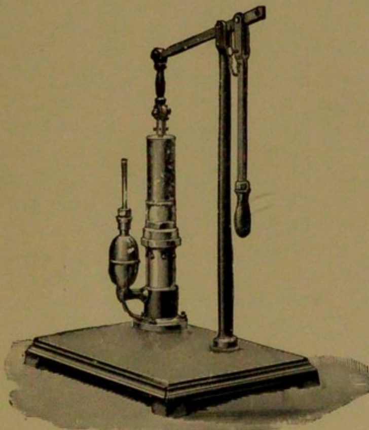
FIG. 35.—Geryk air pump.
