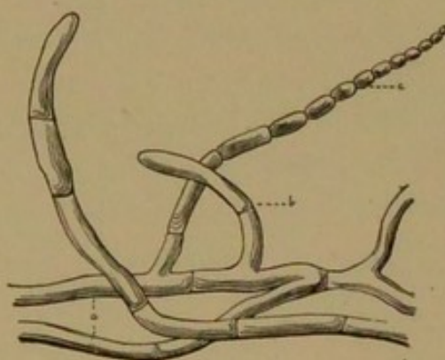
FIG. 80.— Oidium .
