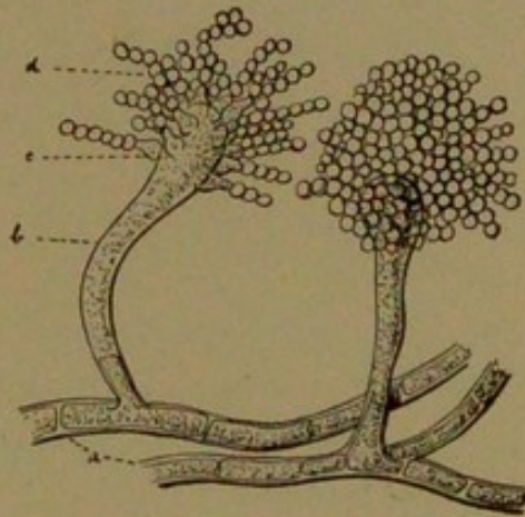
FIG. 78.— Aspergillus
