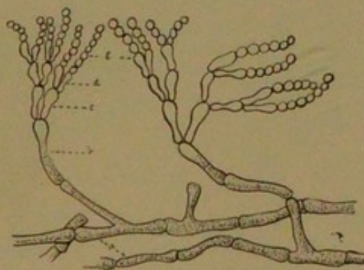
FIG. 79.— Penicillium .
