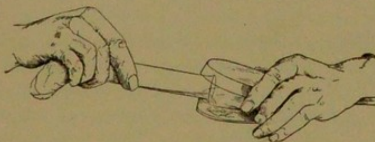
FIG. 125.—Pouring plates.
