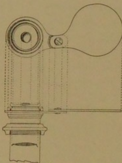
FIG. 49.—Eye shade.
