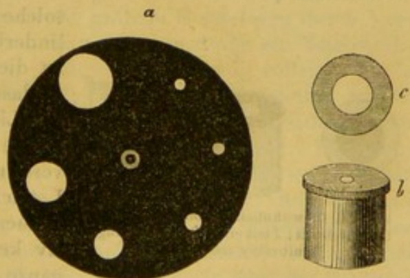
Fig. 22. Diaphragmen. a die Drehscheibe; b, c Zylinderblendungen.
