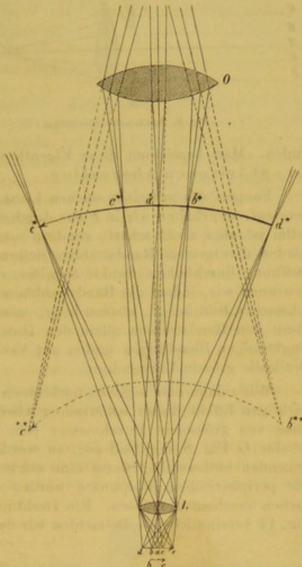
Fig. 8. Das zusammengesetzte Mikroskop in vereinfachter Gestalt.
