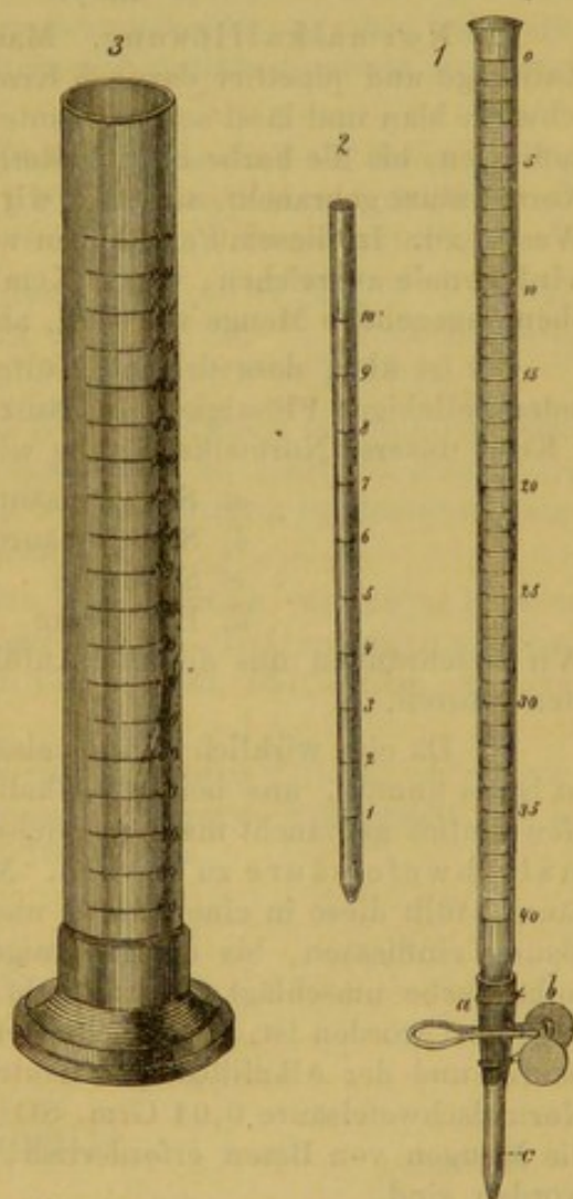
Fig. 61. Titrirapparate. 1 Eine Mohr'sche Bürette mit dem Quetschhahn bei a , der durch Zusammendrücken der beiden Metallknöpfe bei b geöffnet wird und die Flüssigkeit aus der Röhre c austreten lässt; 2 eine Pipette; 3 ein Maasszylinder.
