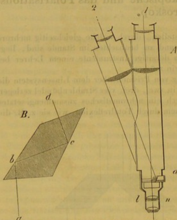
Fig. 36. Wenham's Einrichtung des stereoskopischen Mikroskops.
