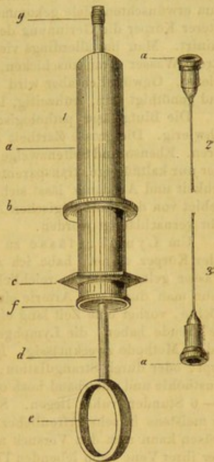
Fig. 65. Die Injektionsspritze 1. a. Die Röhre, mit den vorspringenden Rändern b u. c (zum bequemeren Halten dienend) und dem abzuschraubenden Deckel f; d Stempel mit dem Handgriffe e; g die Oeffnung (Mundstück) der Spritze, von einem Seidenfaden umwickelt. 2 u. 3 Kanülen feinsten Art.
