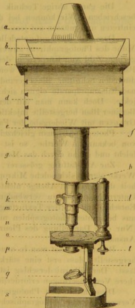
Fig. 33. Gerlach's mikrophotographischer Apparat. a Hohlkegel zum Aufsetzen auf die Visirscheibe; b diese; c Vorsprung oben am Kasten; d Kasten; e Metallring unten an diesem; f Metallring oben am Holzrohr; g dieses; h Metallplatte an dem unteren Ende desselben; i Ring am oberen Ende des Metallrohrs; k Schraube des Metallringes l , welcher zur Verengung der federnden Hülse m dient; n Rohr des Mikroskops mit den Objektiven; o Tisch; p der Metallcylinder zum Tragen von Blende und Beleuchtungslinse; q der Spiegel; r die den Objektisch tragende Metallstange; s das Hufeisen; t die Mikrometerschraube.
