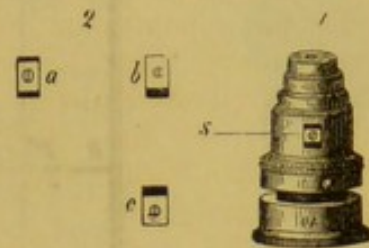
Fig. 19. Achromatisches Linsensystem mit Korrektionsapparat.
