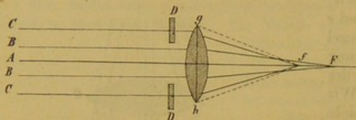
Fig. 9. Sphärische Aberration.
