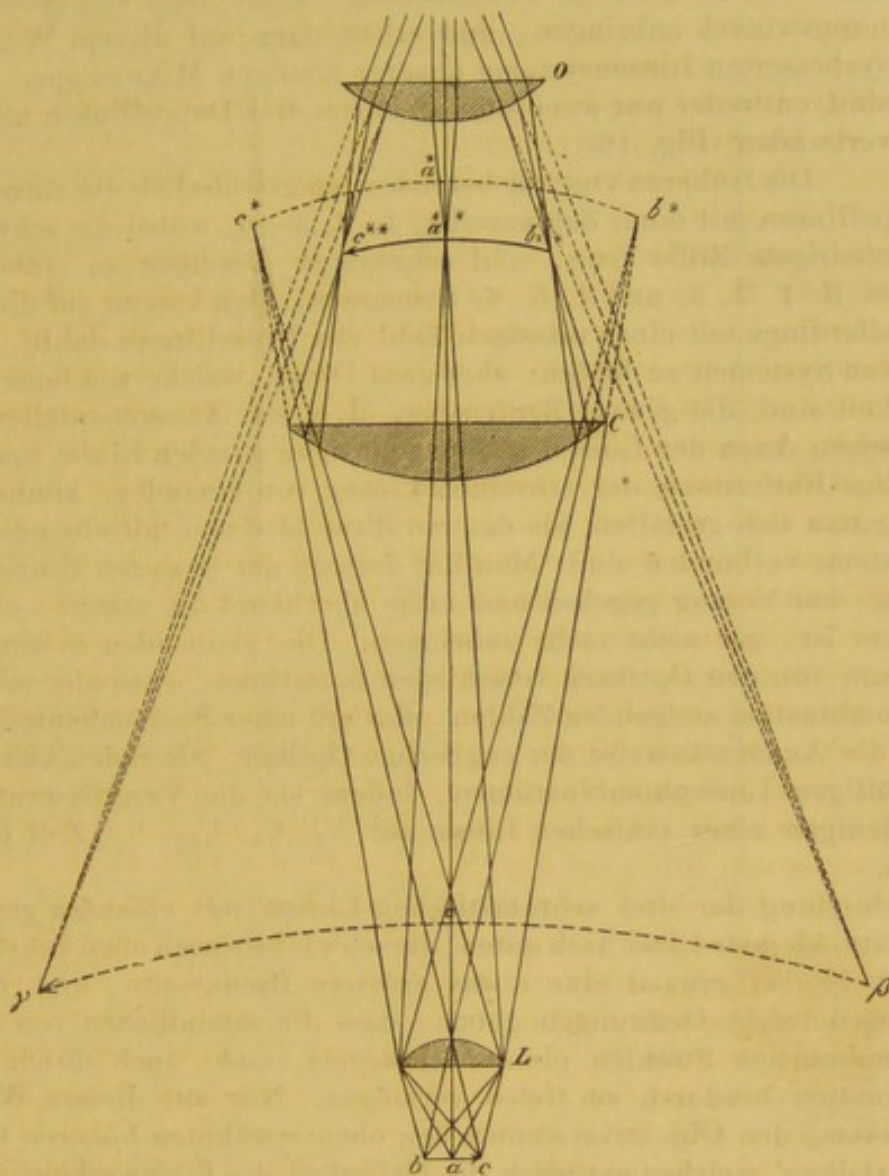
Fig. 15. Das zusammengesetzte Mikroskop mit einer Kollektivlinse.
