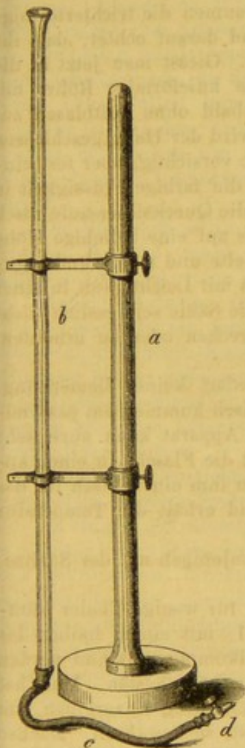
Fig. 62. Einfacher Injektionsapparat mit einer Glasröhre.]
