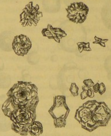
Fig. 232. Krystalle von salpeter- und salzsaurem Xanthin.
