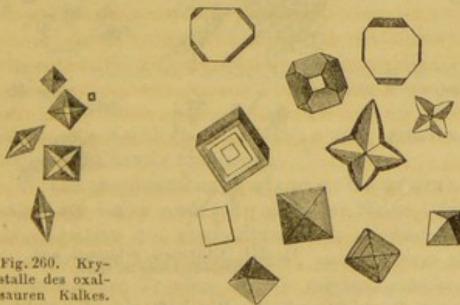
Fig. 261. Verschiedene Krystallformen des Kochsalzes, meistens aus thierischen Flüssigkeiten.
