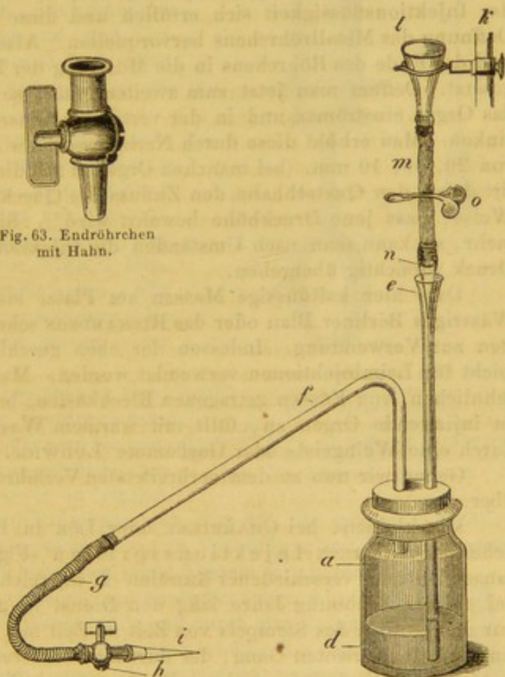
Fig. 64. Injektionsapparat mit einer Quecksilbersäule.
