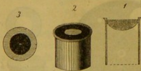
Fig. 24. Gewöhnlicher Kondensor; 1 im Durchschnitt; 2 mit einer Ringblendung; 3 mit einer zentralen.
