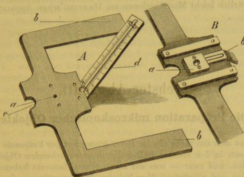
Fig. 54. Erwärmbarer Objektisch von Schultze.
