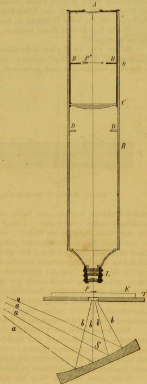
Fig. 17. Das zusammengesetzte Mikroskop.
