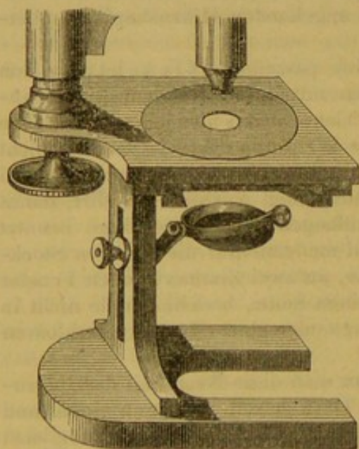
Fig. 52. Schiefe Spiegelstellung am Hufeisenstativ.
