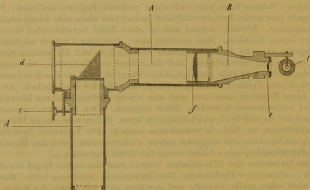
Fig. 32. Camera lucida von Chevalier und Oberhäuser. (Das Stück B ist um 90° gedreht.)
