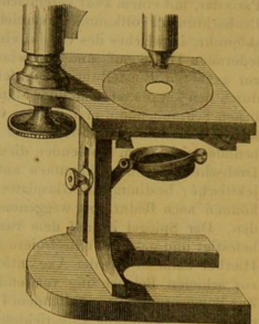
Fig. 28. Dasselbe bei schiefer Beleuchtung.
