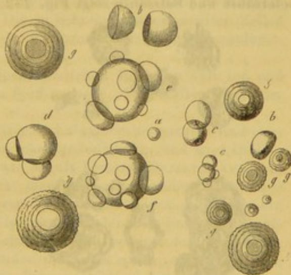
Fig. 230. Verschiedene Krystallmassen des Leucin.
