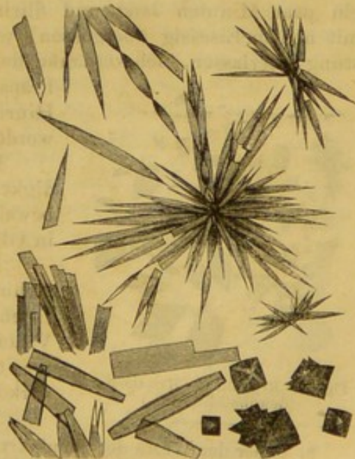
Fig. 80. Krystallformen des Hämatin.
