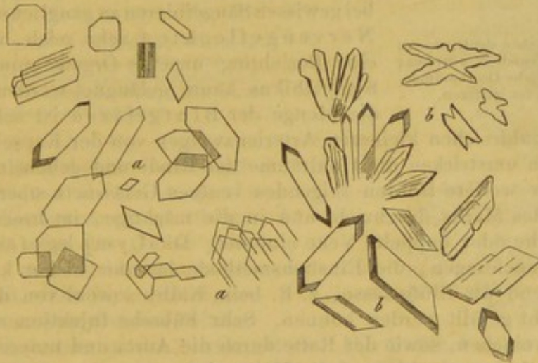
Fig. 266. Krystalle der Verbindungen des Harnstoffs mit Salpetersäure und Oxalsäure. a a Salpetersaurer Harnstoff; b b Oxalsaurer.
