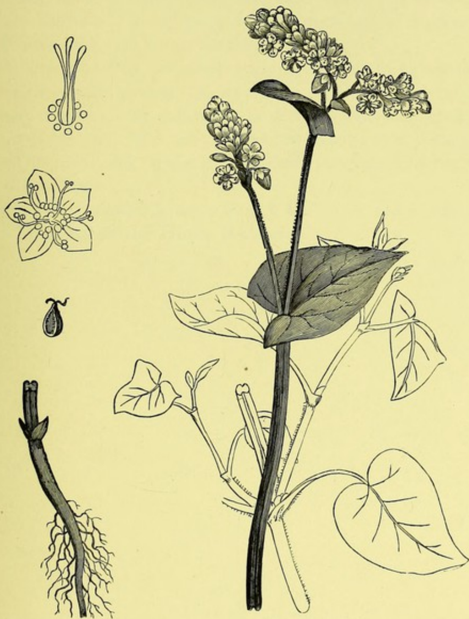
FIG. 21. BUCKWHEAT ( Fagopyrum esculentum ).
