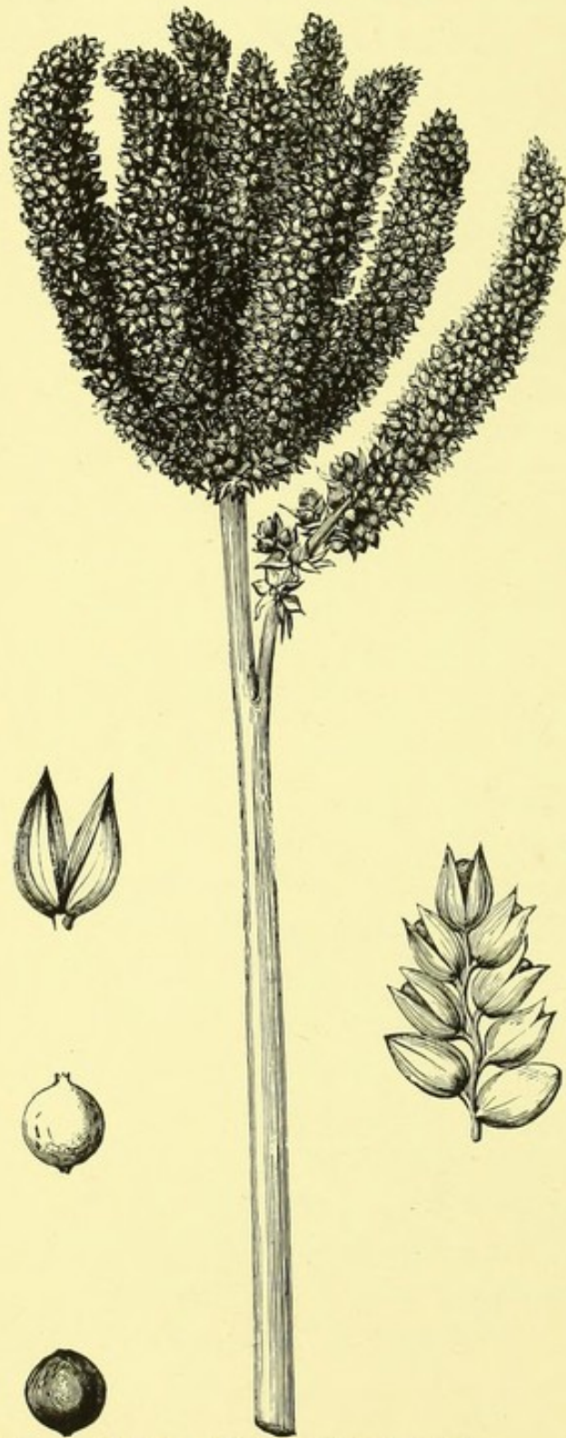
88 FIG. 17. RAGÍ ( Eleusine coracana ).
