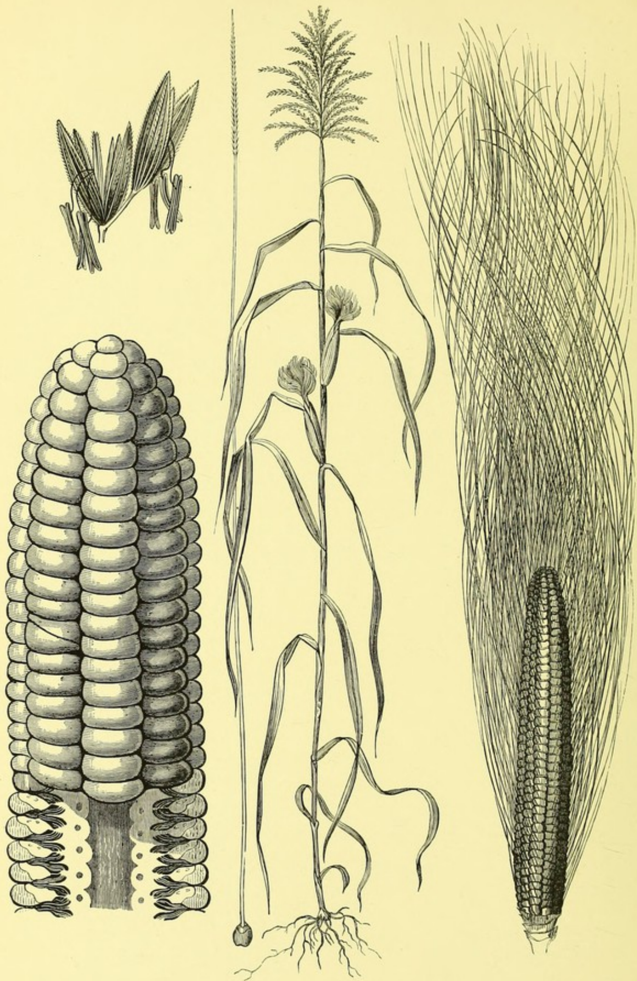
FIG. 11. MAIZE ( Zea Mays ).
