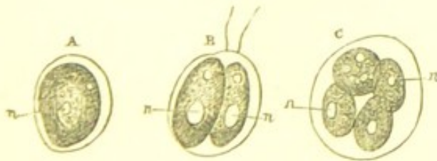
A, B, C. Multiple fission of Chlamydomonas . n. Nuclei.
