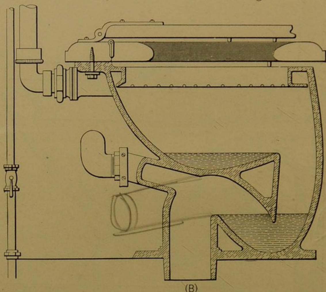
FIG. 5b.—Wash-out Closet.
