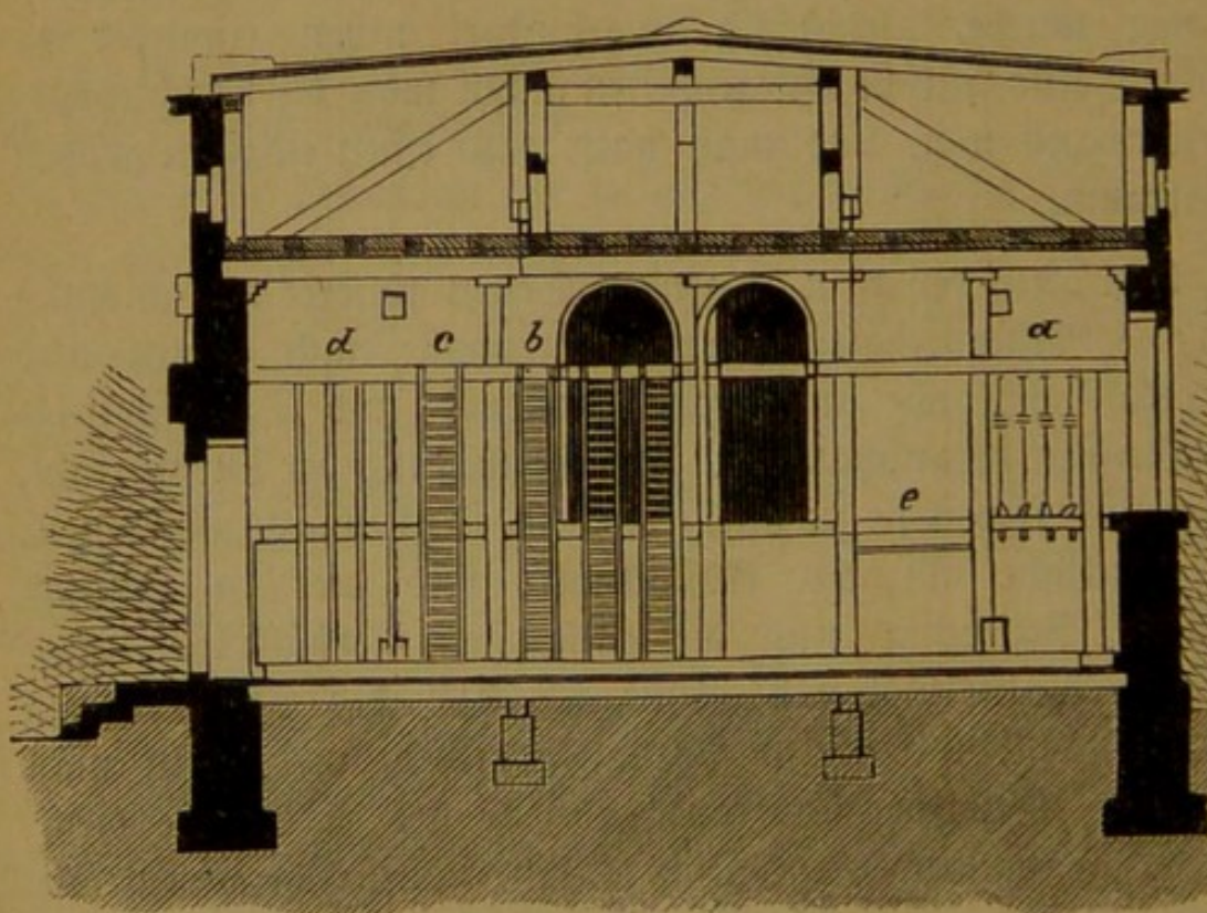
Turnhalle: Durchschnitt.
