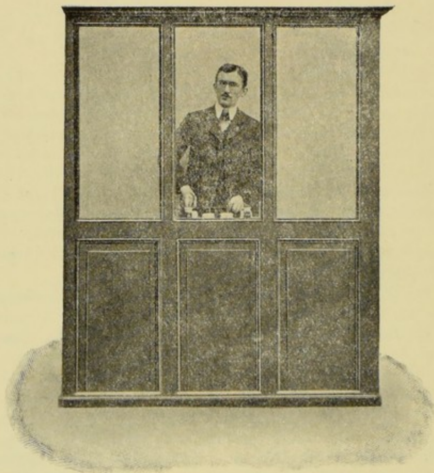
Figur 73. Schutzhaus von vorn mit Reguliertisch.
