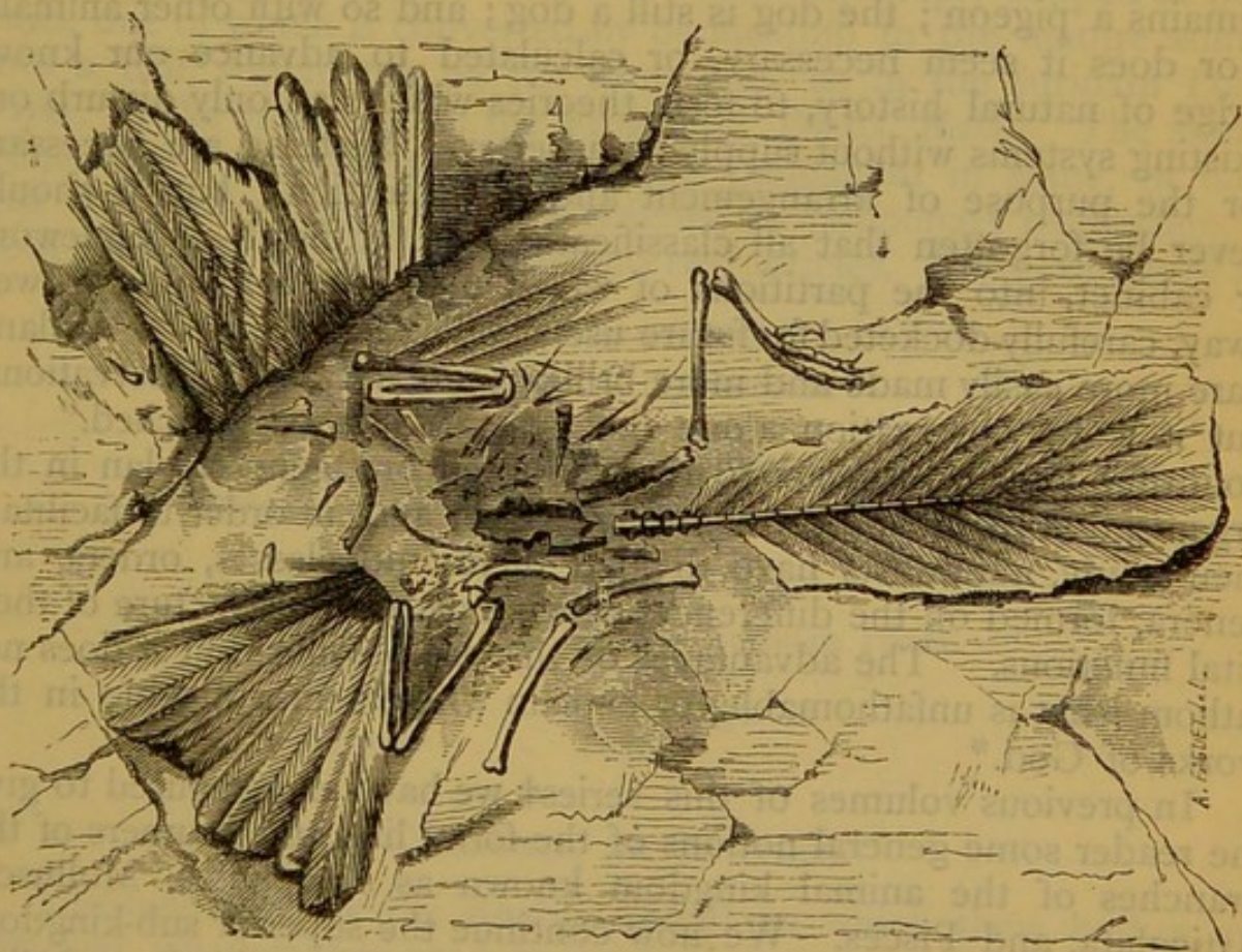
Fig. 1.—Archæopteryx lithographicus.
