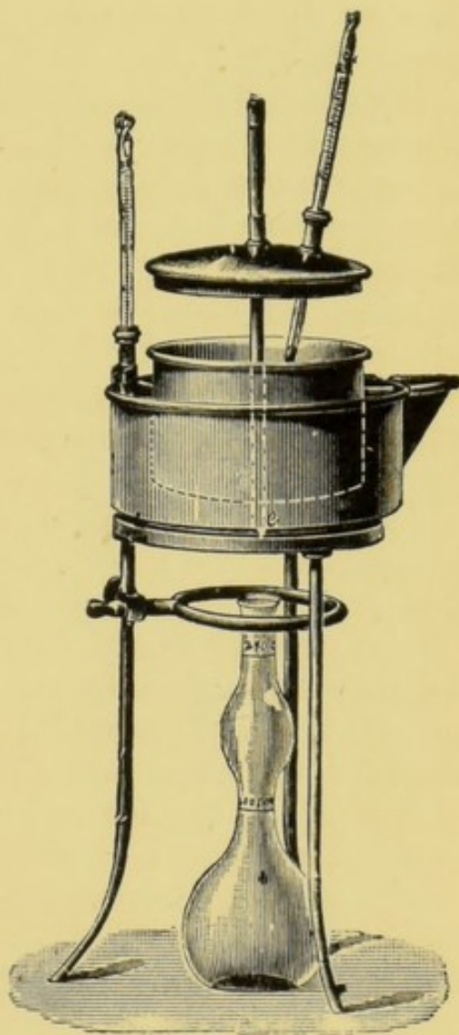
FIG. 16.—Engler Viscometer.
