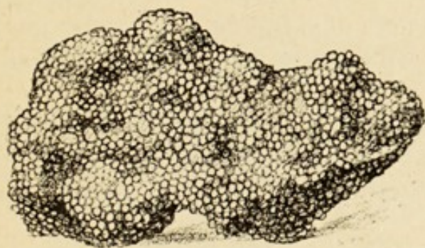
FIG. 201. — Calcaire oolithique .
