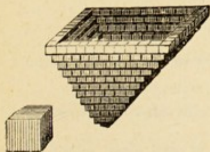
FIG. 205. — Sel gemme en trémie et en cube.
