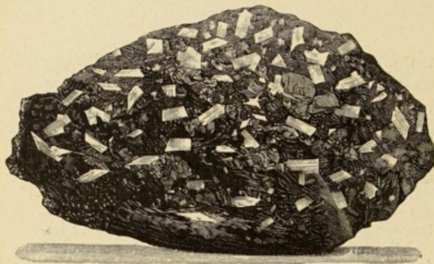
FIG. 208. — Porphyre.
