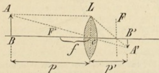
FIG. 139. — Construction de l'image A'B' d'un objet AB , donnée par la lentille L .
