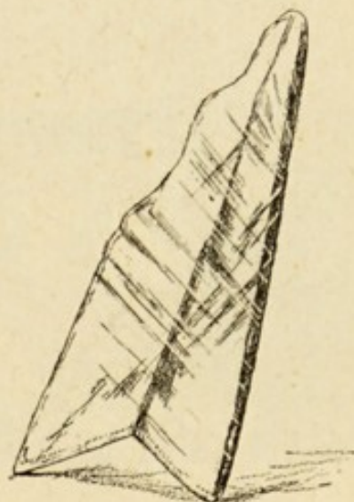
FIG. 204. Gypse en fer de lance.
