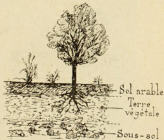
FIG. 178. — Le sol comprend le sol arable et la terre végétale, reposant sur le sous-sol.
