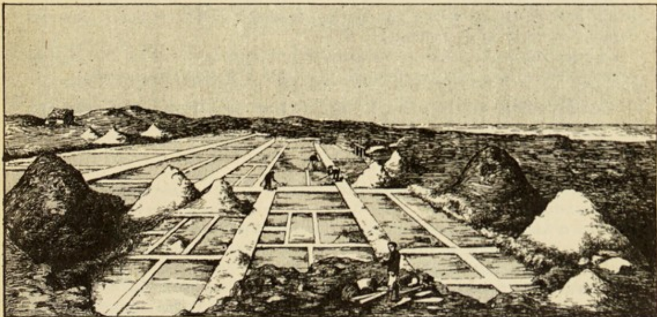
FIG. 37. — Marais salants.
