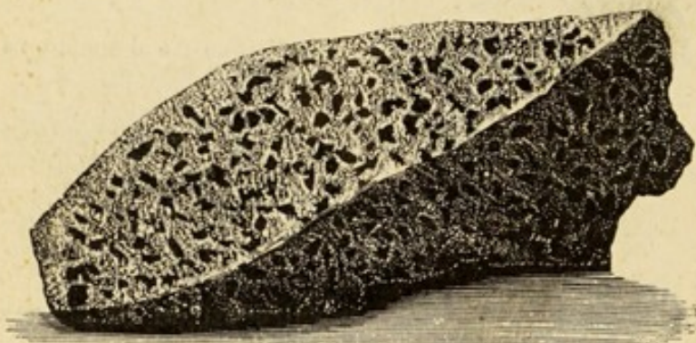
Fig. 207. — Granite (les parties noires représentent les cristaux de mica non orientés).
