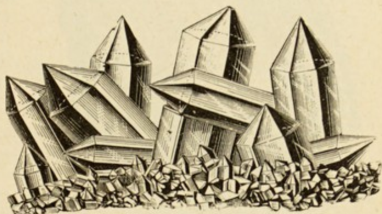
FIG. 187. — Groupe de cristaux de quartz.
