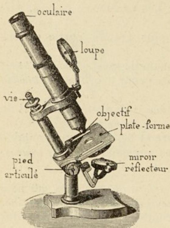
FIG. 34. — Le microscope.
