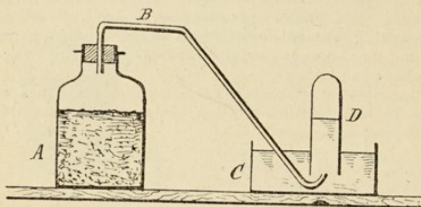
FIG. 13. — Fermentation alcoolique.
