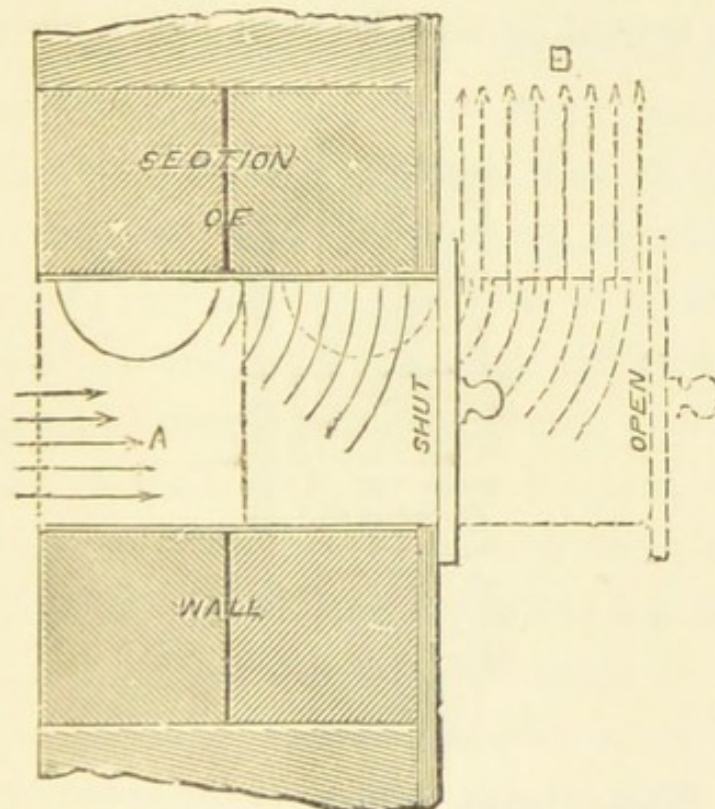
FIG. 6.—Drawer Ventilator.
