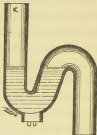
FIG. 44.—Lead siphon trap.
