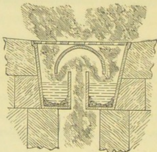
FIG. 30.—Bell-trap.
