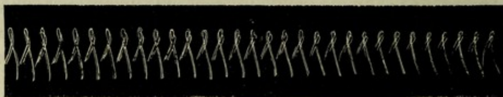
Fig. 79. — Graphique d'une verge de Wheatstone accordée à l'octave, munie d'une aile de guêpe et orientée de manière à enregistrer surtout la boucle supérieure du 8.
