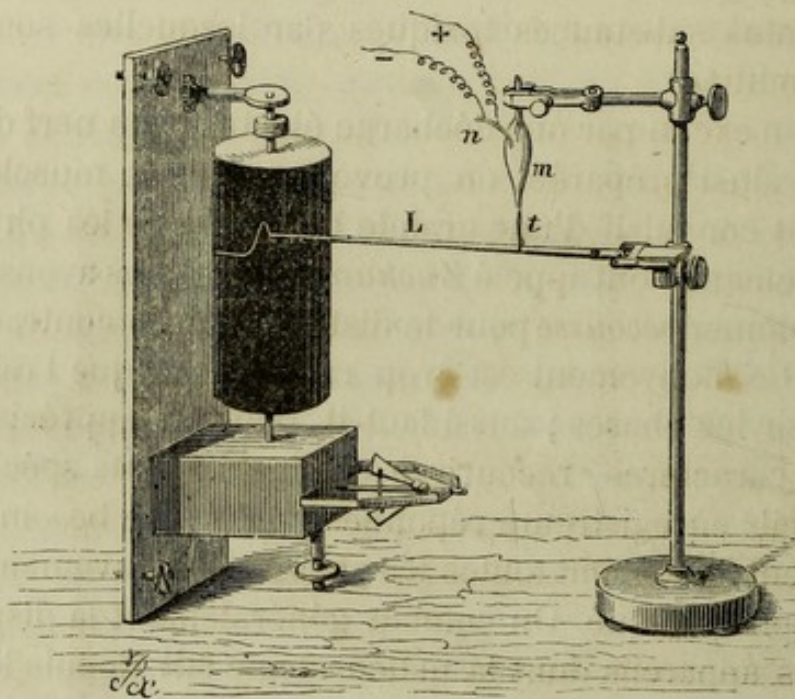
Fig. 2. — Description théorique du myographe.
