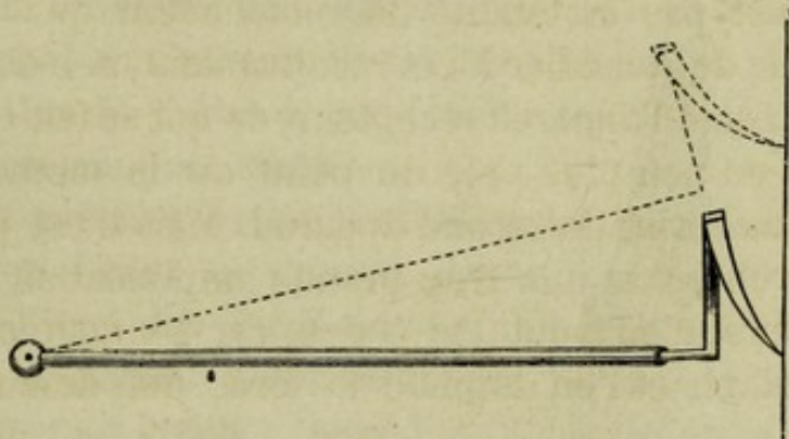
Fig. 98. — Pointe élastique traçant sur une glace enfumée.
