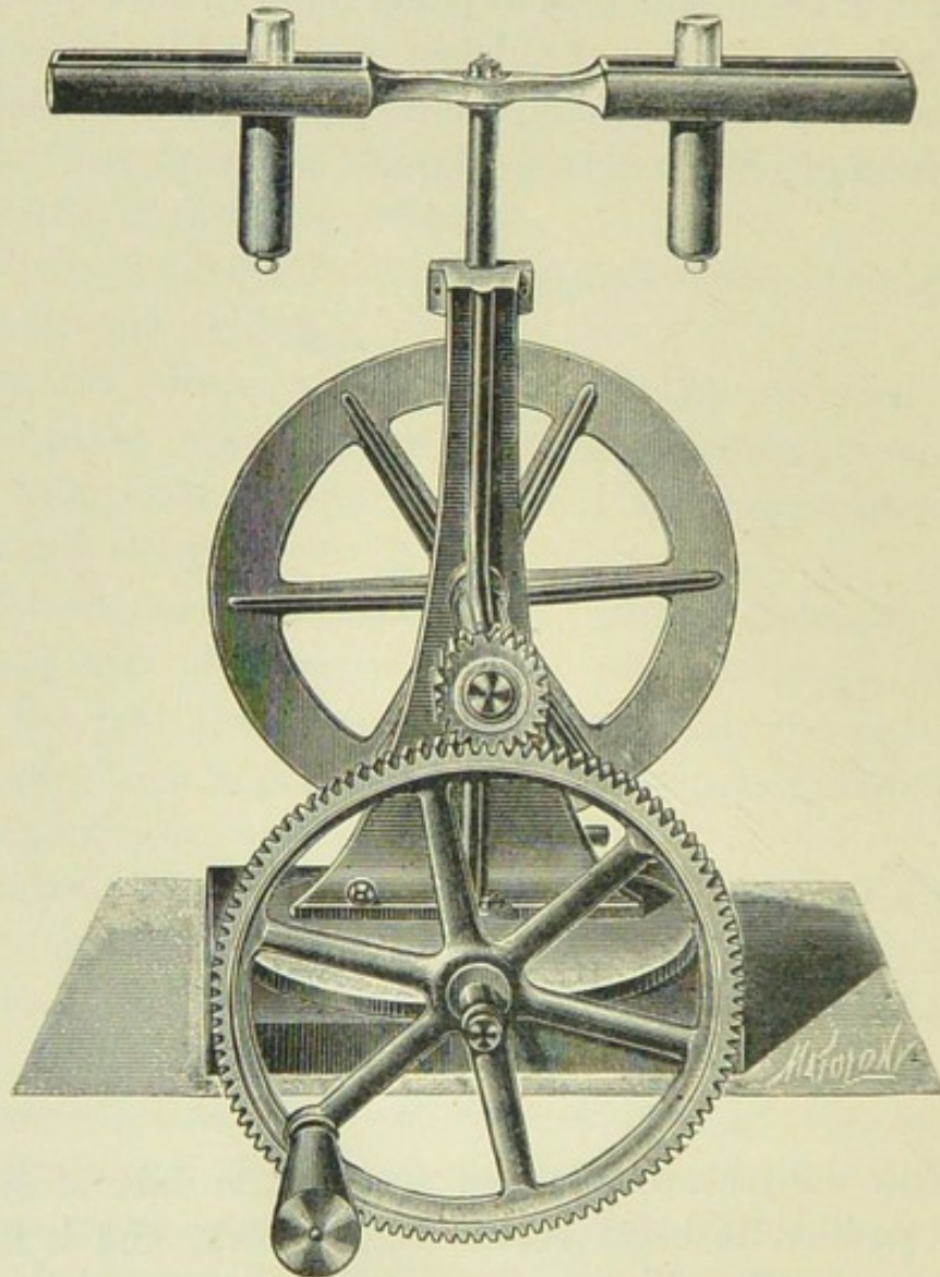
FIG. 20.—STENBECK'S CENTRIFUGE (after Jaksch).
