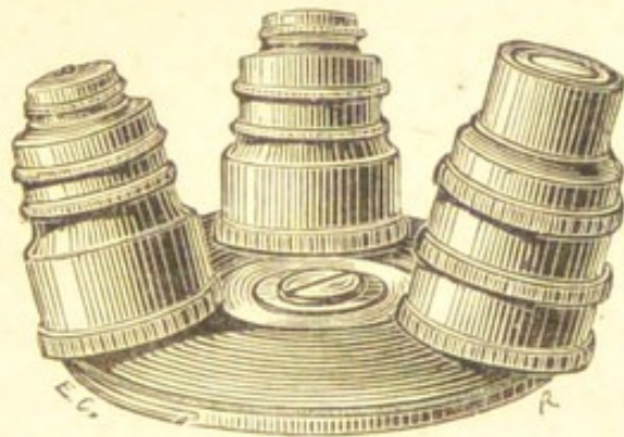
Fig. 11. — Revolver à trois objectifs (vu renversé) ; un quatrième objectif peut être adapté à la place restée vide (en avant).
