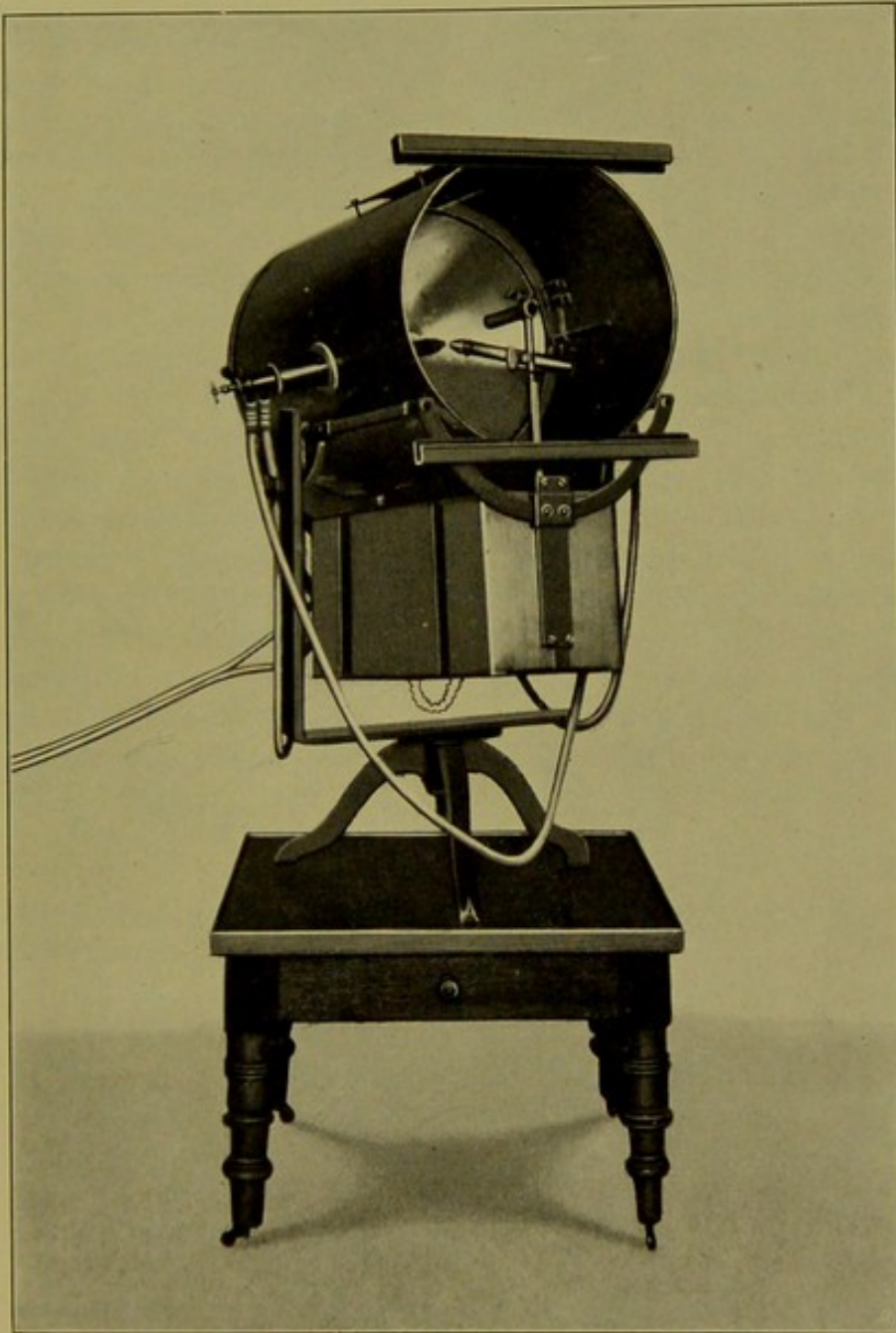
Bogenlampe mit wassergekühlten Eisenelectroden.
