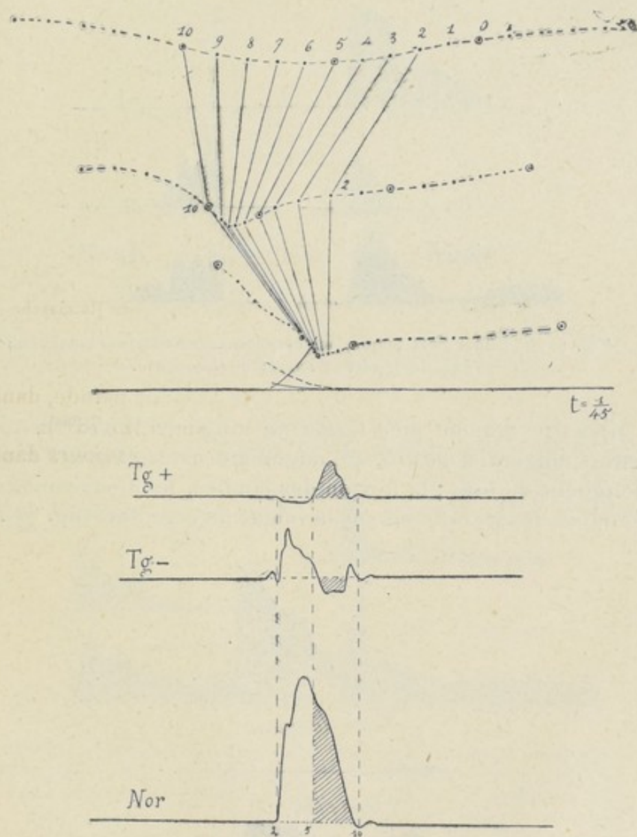
FIG. 80. — Mouvement de la jambe et pressions normale et tangentielles du pied sur le sol pendant un appui du pied dans la course. Les chiffres indiquent des \frac{1}{45} de seconde.
