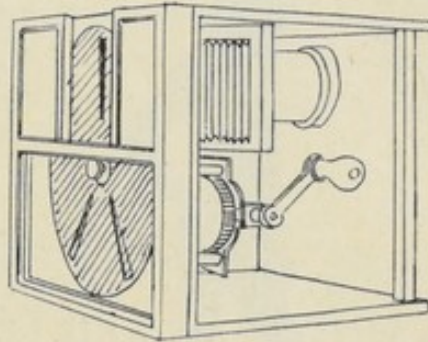
FIG. 61. — Appareil chronophotographique de Marey.
