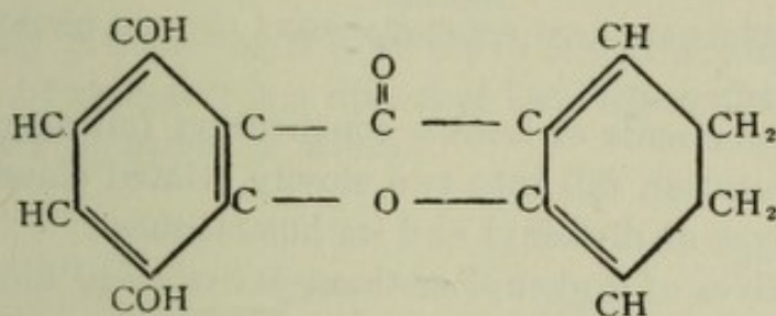
Rhamnocitrin
