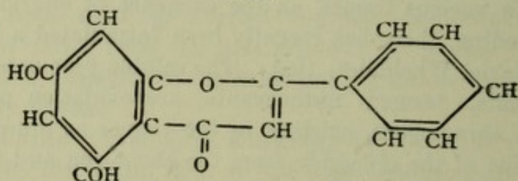
flavone
