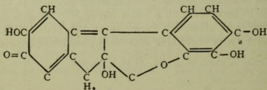
Haematein
