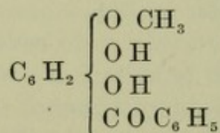
Cotoin.
