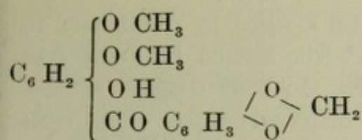
Protocotoin.
