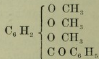
Methyl hydrocotoin
