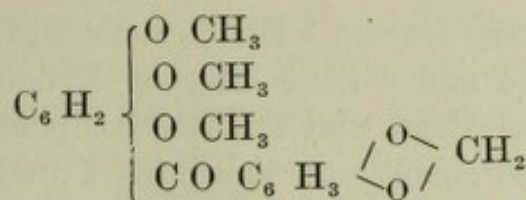
Methyl protocotoin.
