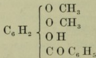
Hydrocotoin
