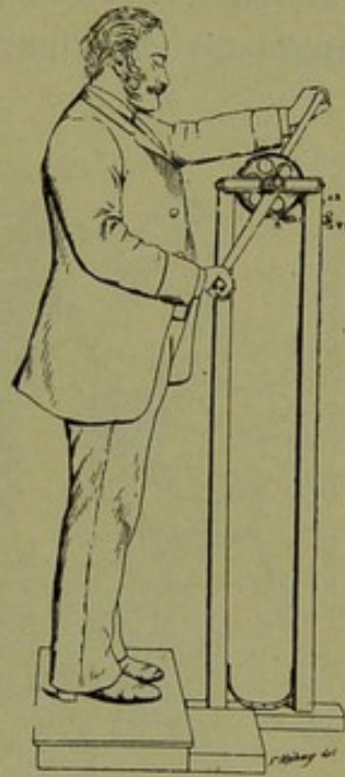
Fig. 21. — Appareil de Nycander pour exercer les muscles des bras. — (La résistance est obtenue au moyen d'une lame métallique enroulée autour de la roue R et qu'on serre à volonté à la manière d'un frein, au moyen d'une vis de tension V. T.)
