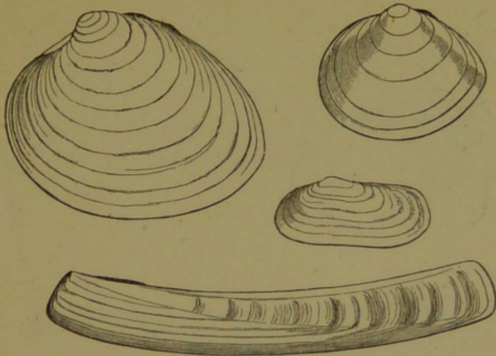
ACEPHALA.
