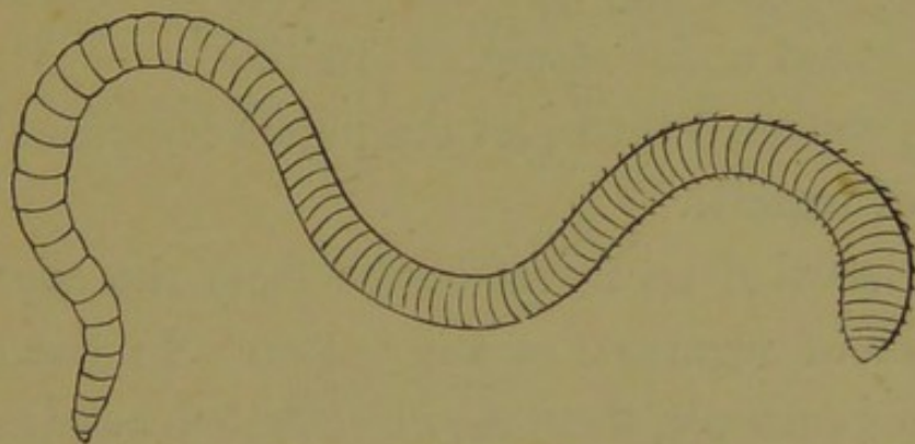
FIG. 82.—EARTHWORM.
