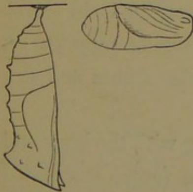
FIG. 72.—CHRYSLIDES.
