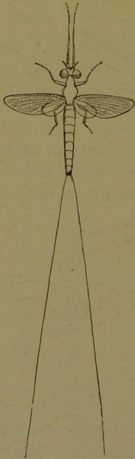
FIG. 98.—EPHEMERA.
