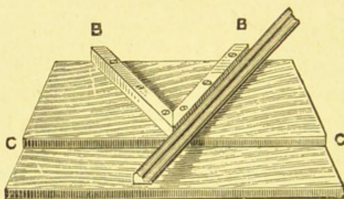
FIG. 40.—MITRE BLOCK.
