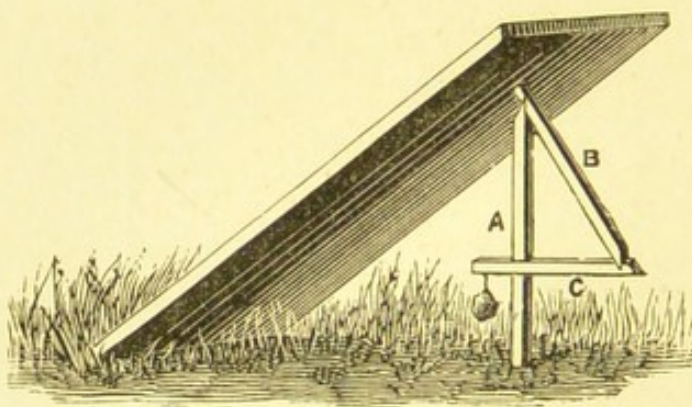
FIG. 4.—"FIGURE OF 4" TRAP.
