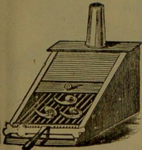
Gril fumivore.
