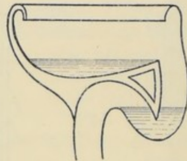
FIG. 94.—Wash-out closet.
