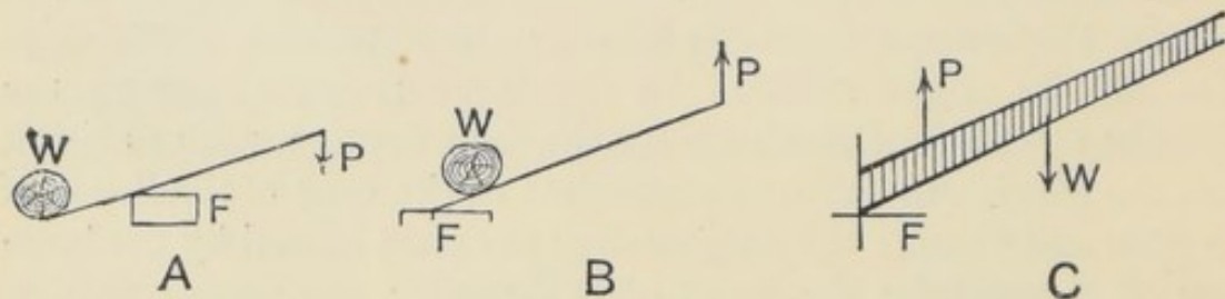
FIG. 18.—Levers.
