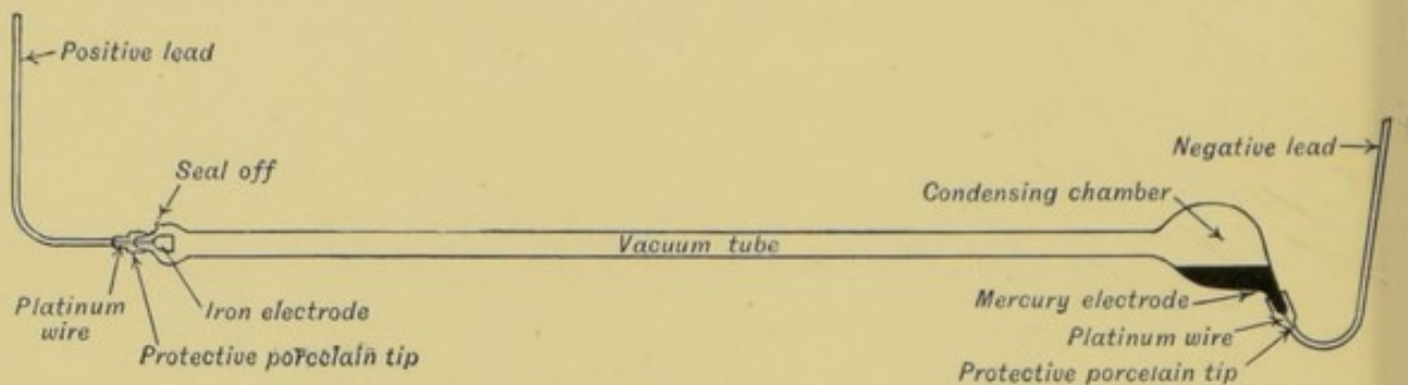
FIG. 200.—Cooper-Hewitt Mercury Vapour-lamp.
