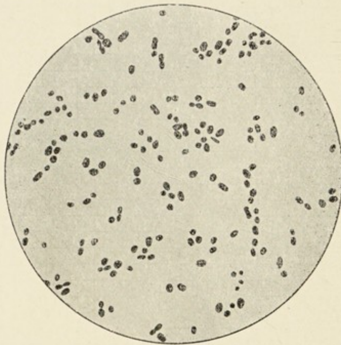
BACILLUS PESTIS.
