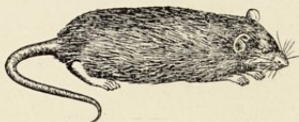
NESOKIA BENGALENSIS.
