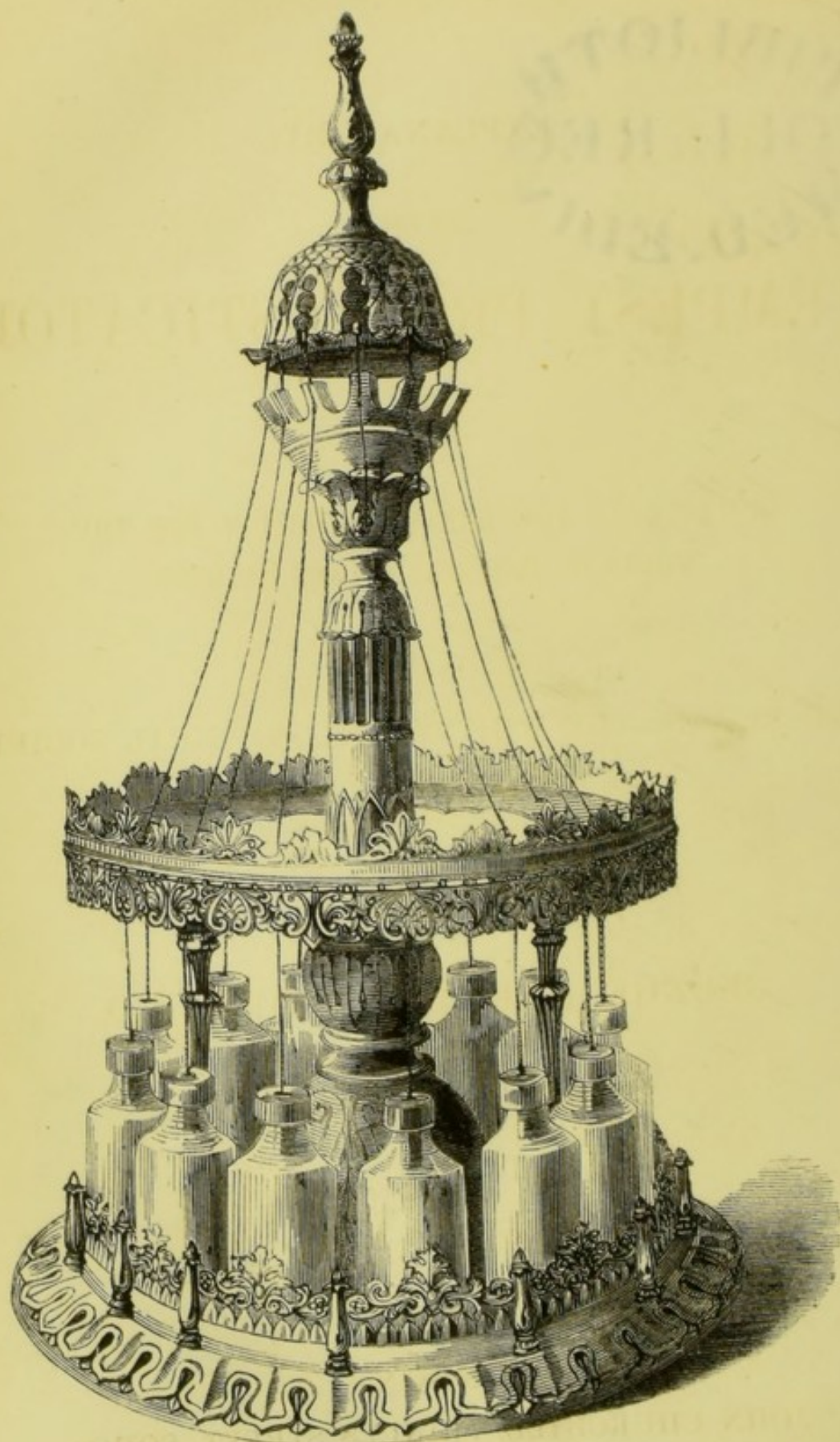
TEMPEST PROGNOSTICATOR.
