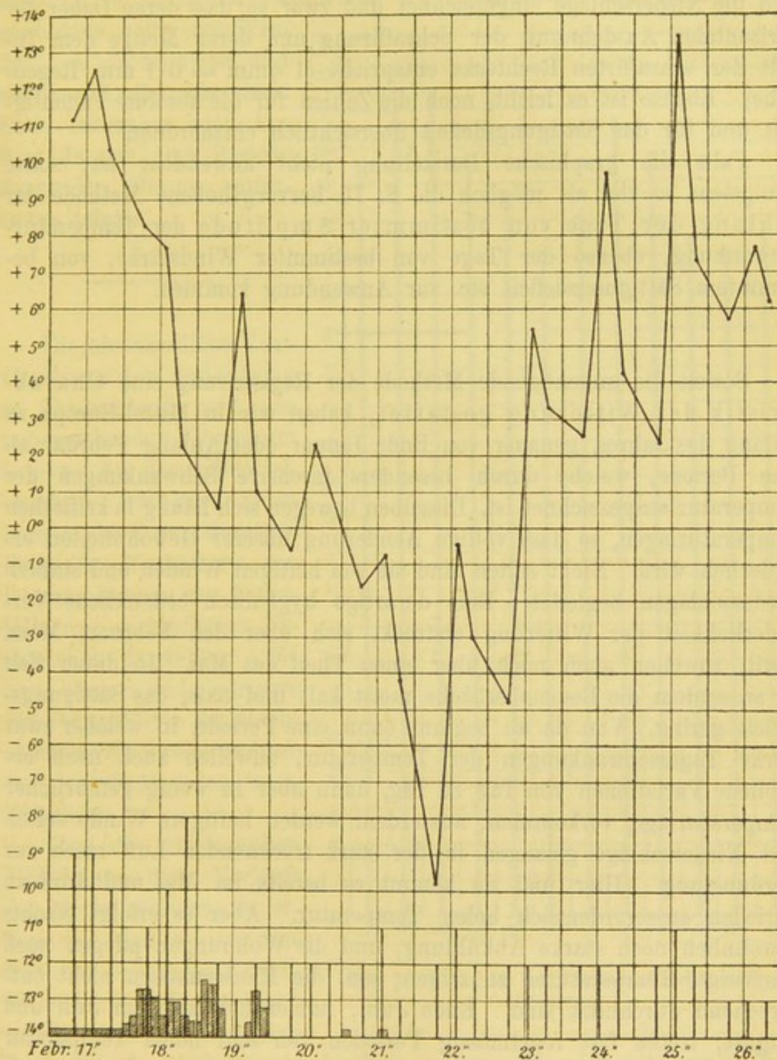
Fig. 1. Witterung vom 17.—26. Februar 1885.
