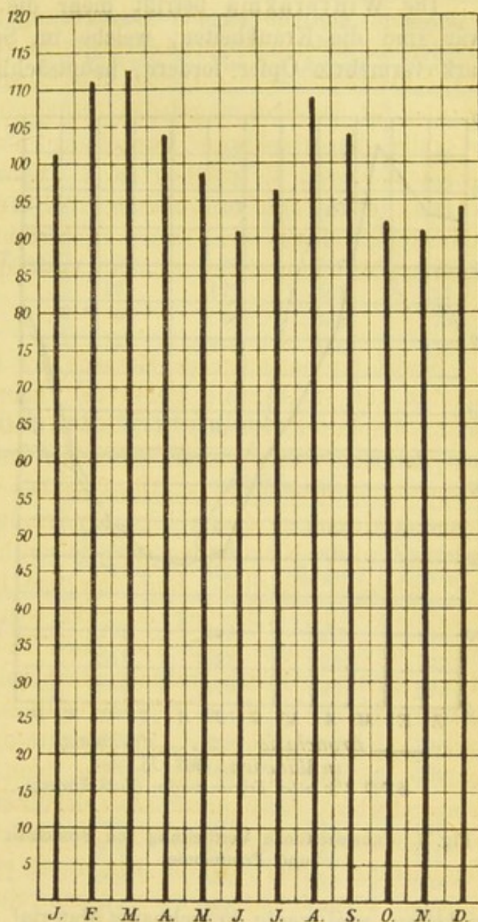
Fig. 2. Mortalität im Deutschen Reich nach Monaten.
