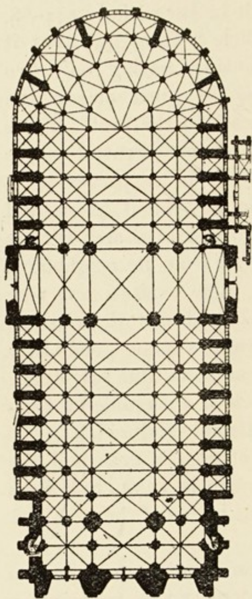
FIG. 90. Plan of Notre Dame, Paris.
