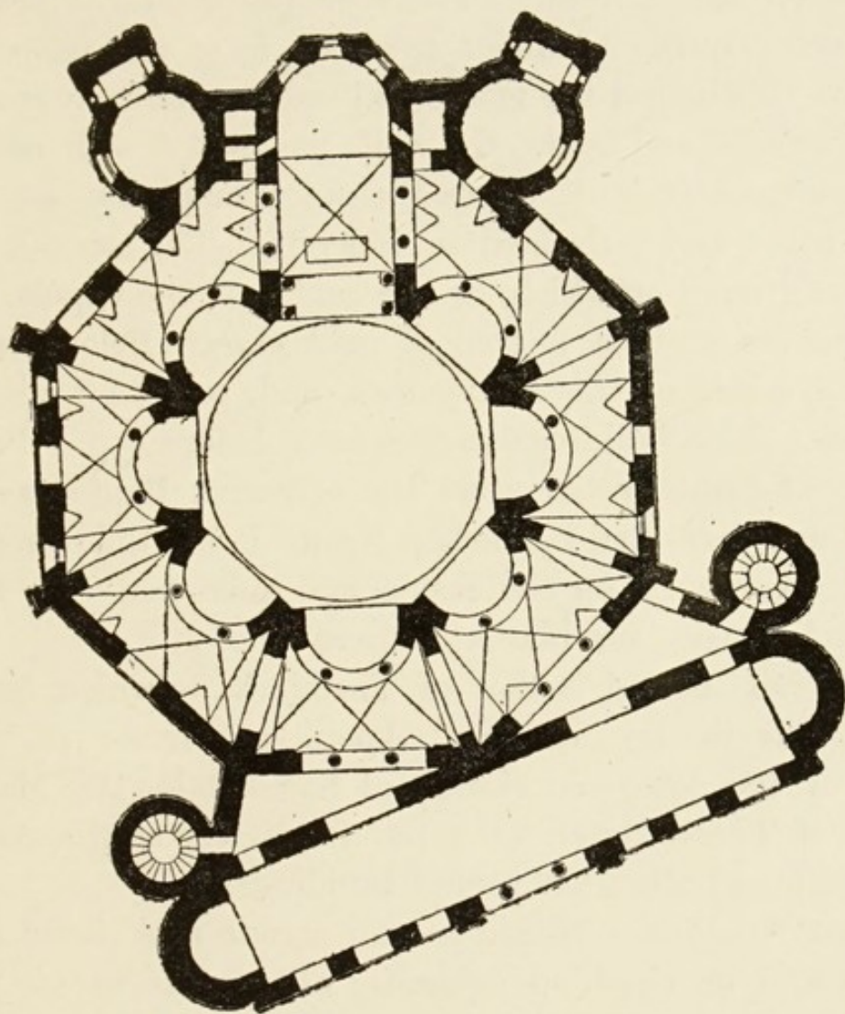
FIG. 28. Plan of St. Vitale, Ravenna.
