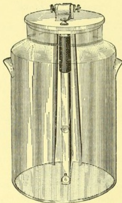
FIG. 1.—Edison-Lelande cell, type W.
