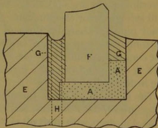
FIG. 3.—Bottom edge glass on aquarium fronts, Monaco.
