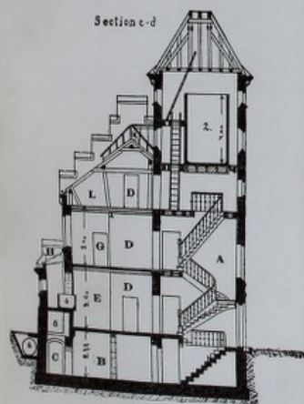
FIG. 5.—SECTION AT c-d (FIG. 1).
