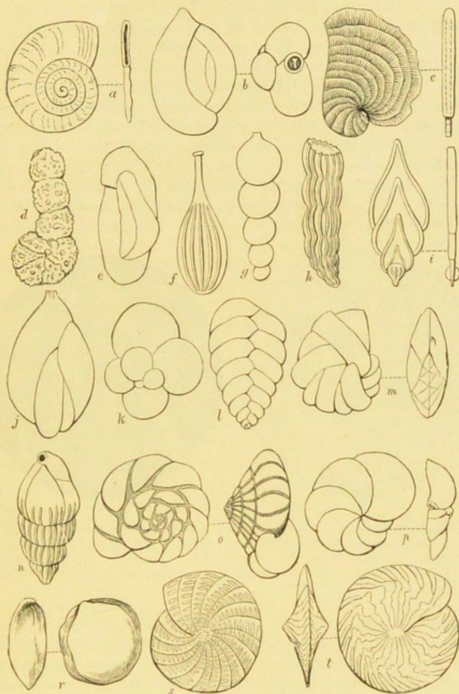
FIG. 3.—Examples of Foraminifera:—
