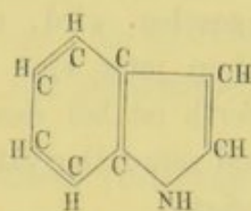
Indol.
