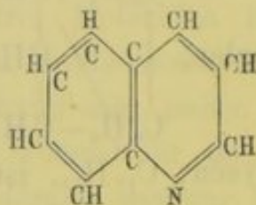
Chinolin.
