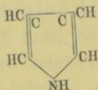
Pyrrol
