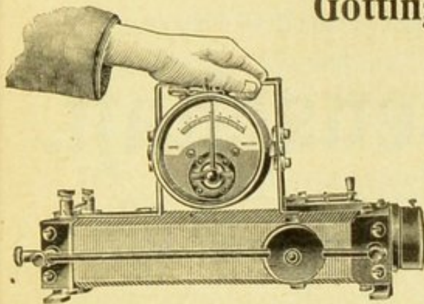
Universal-Abzweig-Widerstände von Mk. 30.— bis Mk. 45.— mit Meßinstrument Mk. 30.— mehr.
