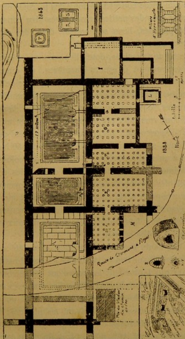
Fig. 48. — PLAN DES THERMES GALLO-ROMAINS DE ROYAT.
