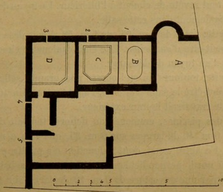
Fig. 46. — PLAN DES THERMES DE SAINT-GALMIER.
