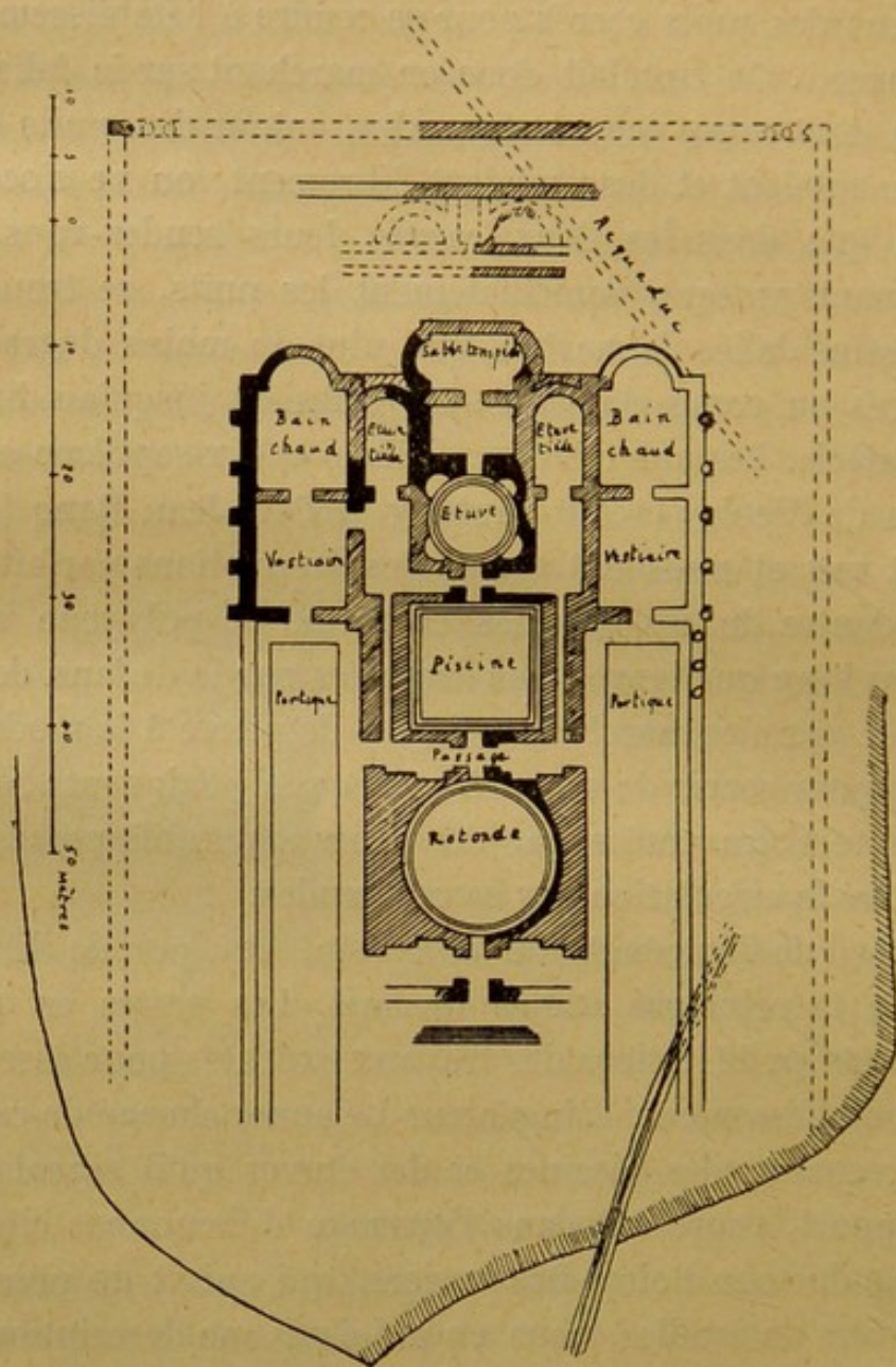
Fig. 58. — PLAN DU PREMIER ÉTABLISSEMENT DE NÉRIS. D'après le plan d'Esmonnot.
