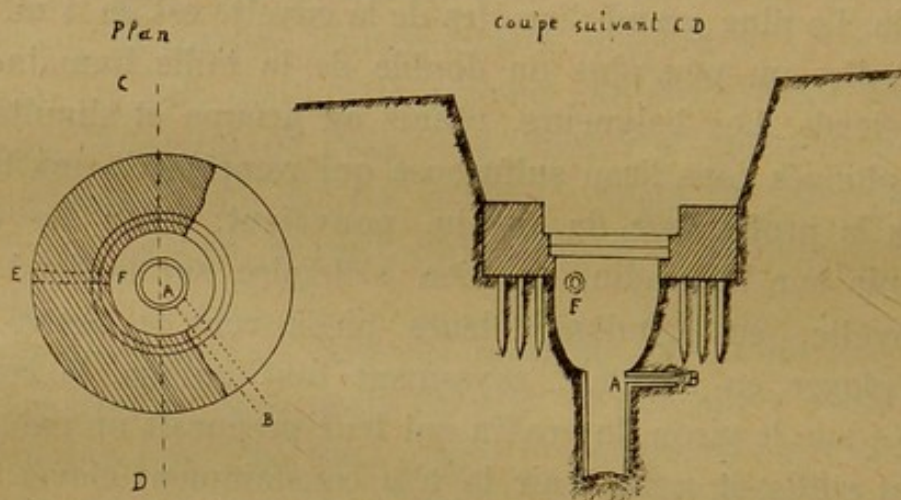
Fig. 44. — Puits de la source des Fumades.
