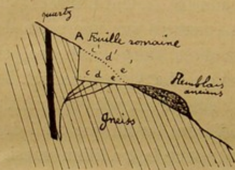
Fig. 54. — COUPE THÉORIQUE DU CAPTAGE ROMAIN A ÉVAUX.
