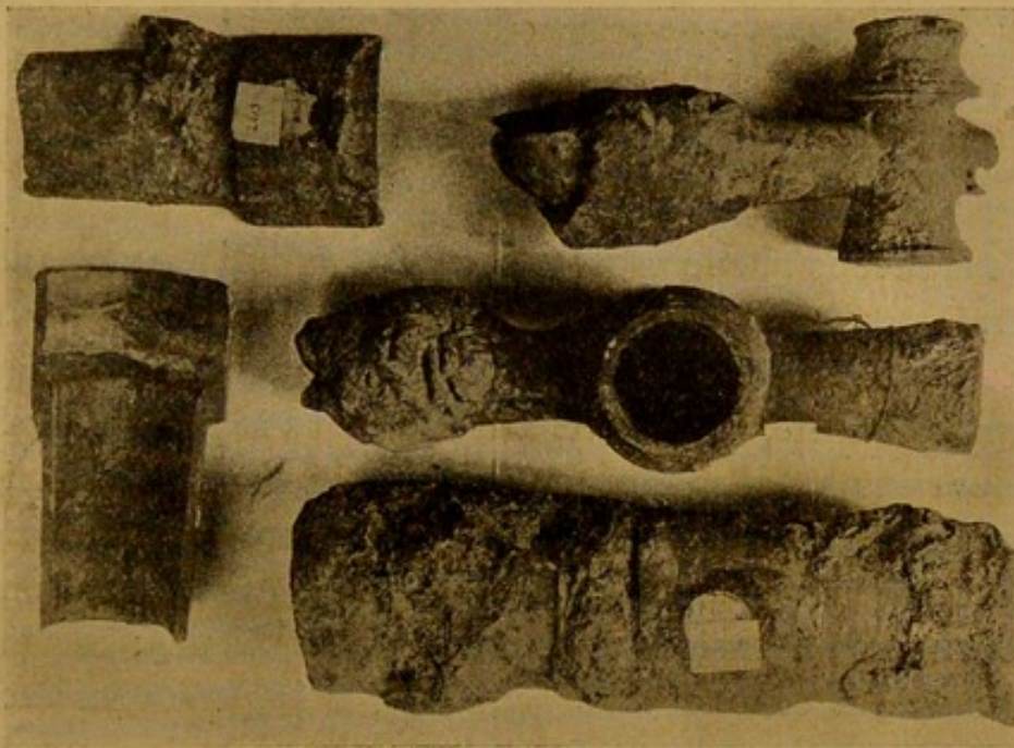
Fig. 72. — ROBINETS ET SECTIONS DE TUYAUX DE BOURBONNE, CONSERVÉS AU CABINET DES ANTIQUES.
