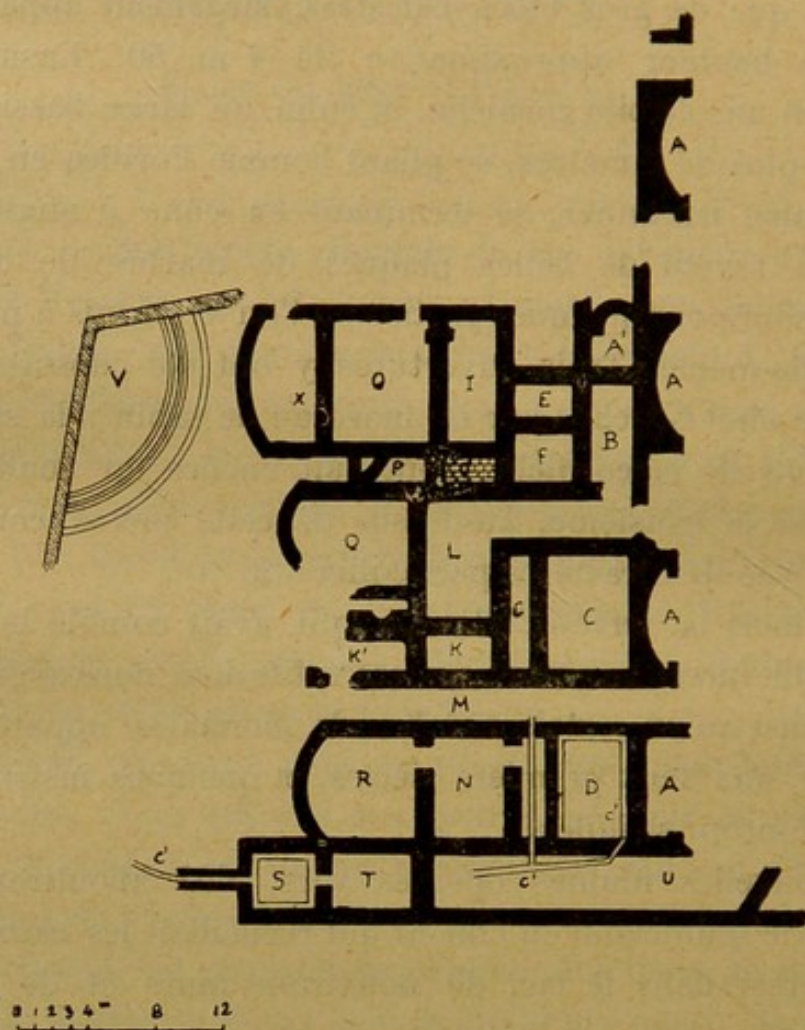
Fig. 38. — PLAN DES THERMES DE MENTHON.
