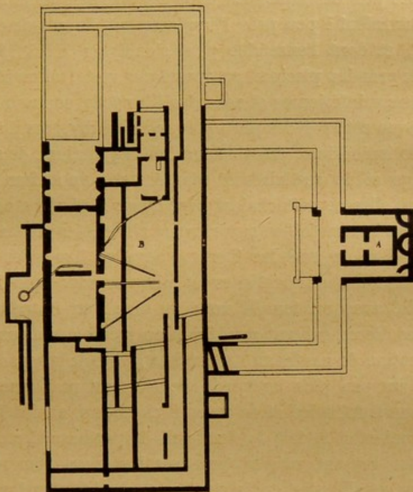
Fig. 50. — PLAN DES THERMES GALLO-ROMAINS DU MONT-DORE.
