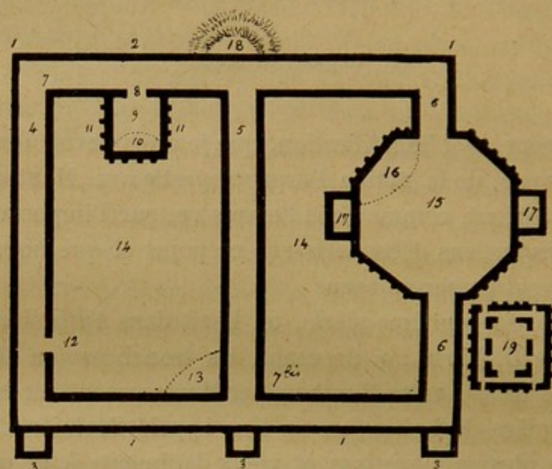
Fig. 68. — PLAN DES THERMES DE MONTBOUY.
