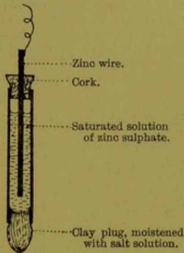
FIG. 7.—NON-POLARISABLE ELECTRODE.
