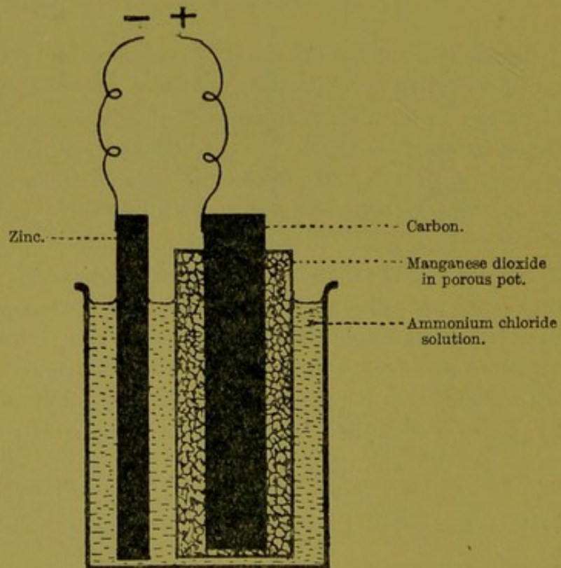
FIG. 4.—LECLANCHÉ CELL.
