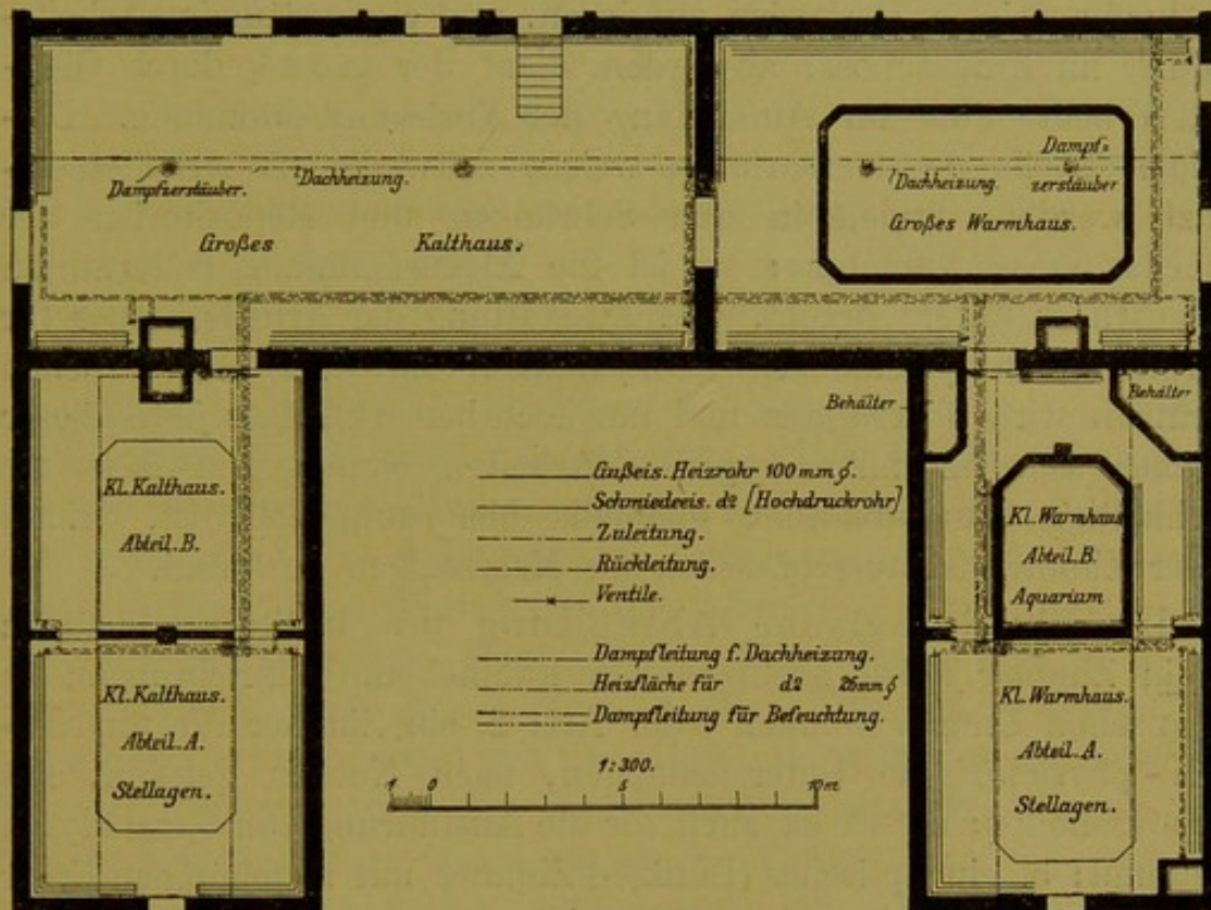
Heizungsanlagen der Gewächshausbauten.
