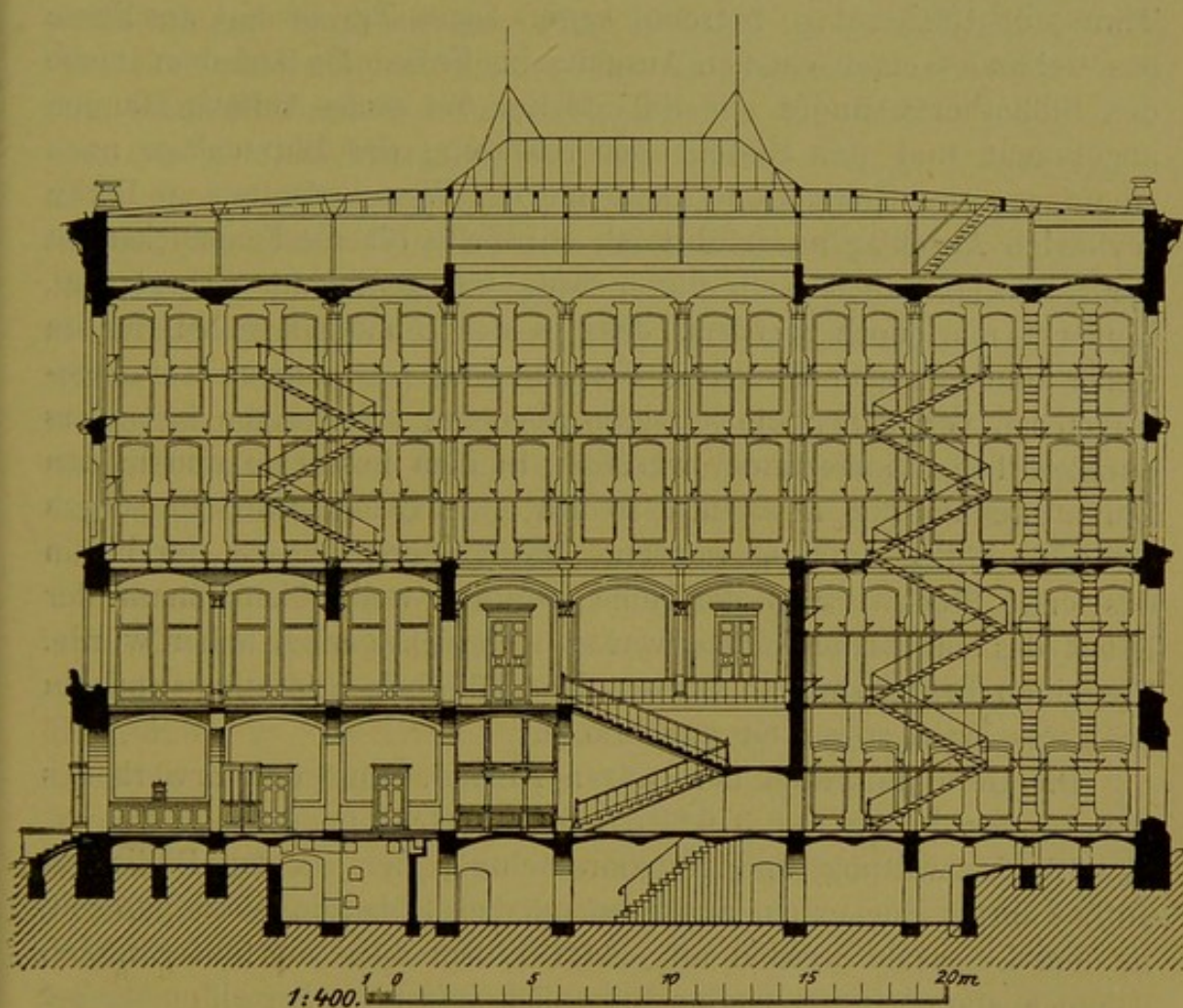
Querschnitt.
