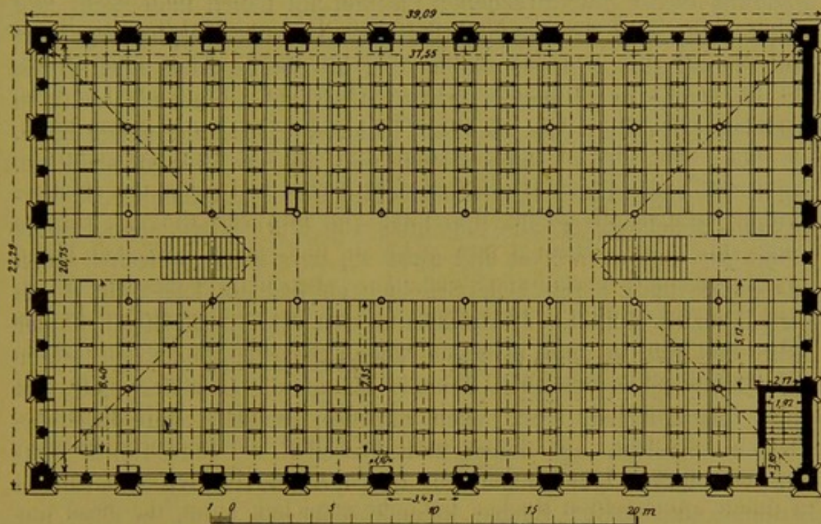
Die eisernen Zwischendecken der oberen Bücheretagen.
