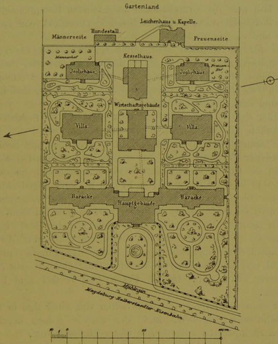
Lageplan.
