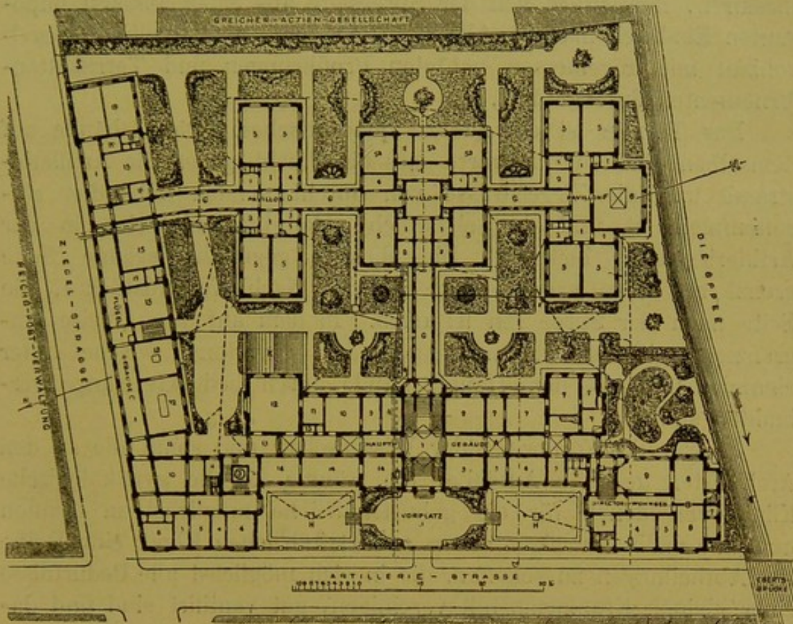
Lageplan.
