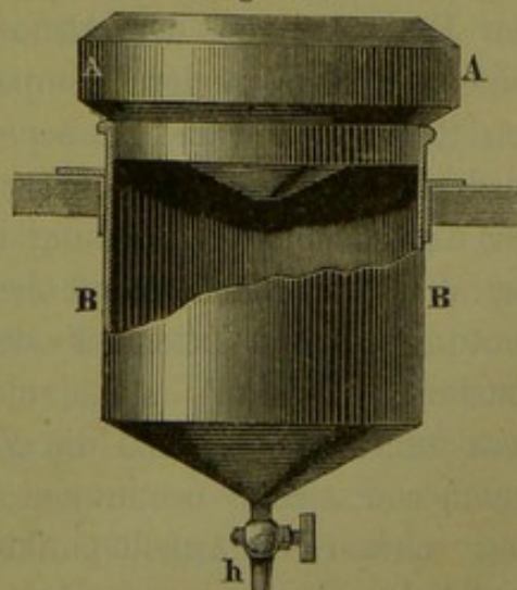
Regenmesser. Auffanggefäss.
