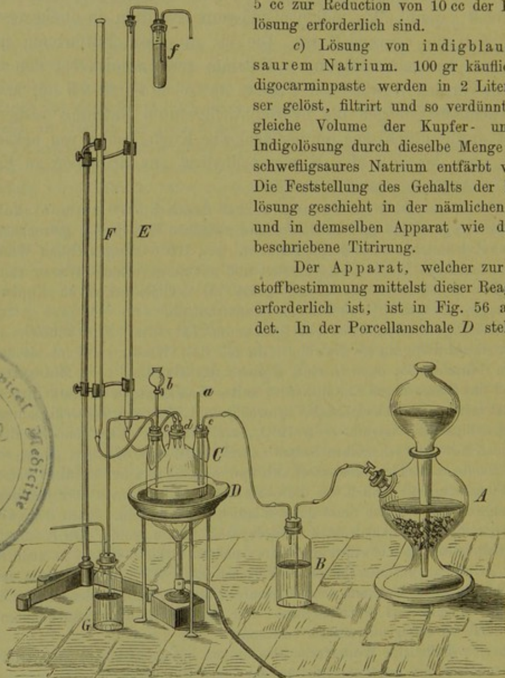
Apparat zu SCHÜTZENBERGER und RISLER's Sauerstoffbestimmung.
