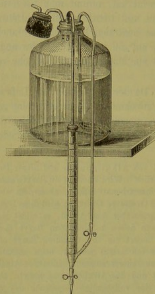
Aufbewahrung der Titirlösung.
