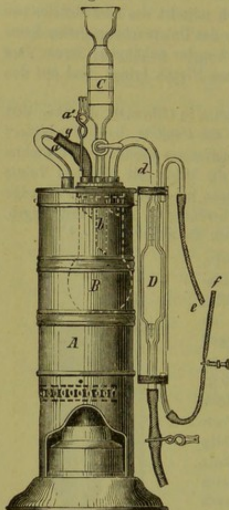
Apparat zur Wasserbestimmung in der Milch.
