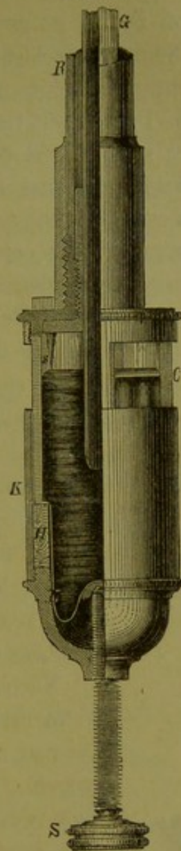
Barometer nach Fortin. Unterer Theil.
