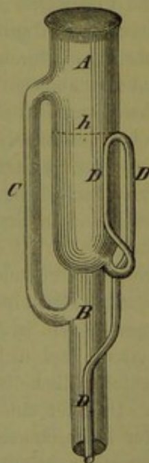
Fettextractions-Apparat von Soxhlet.
