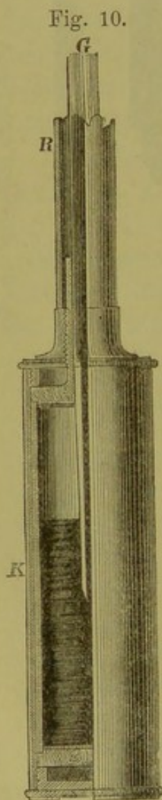
Stationsbarometer. Unterer Theil.
