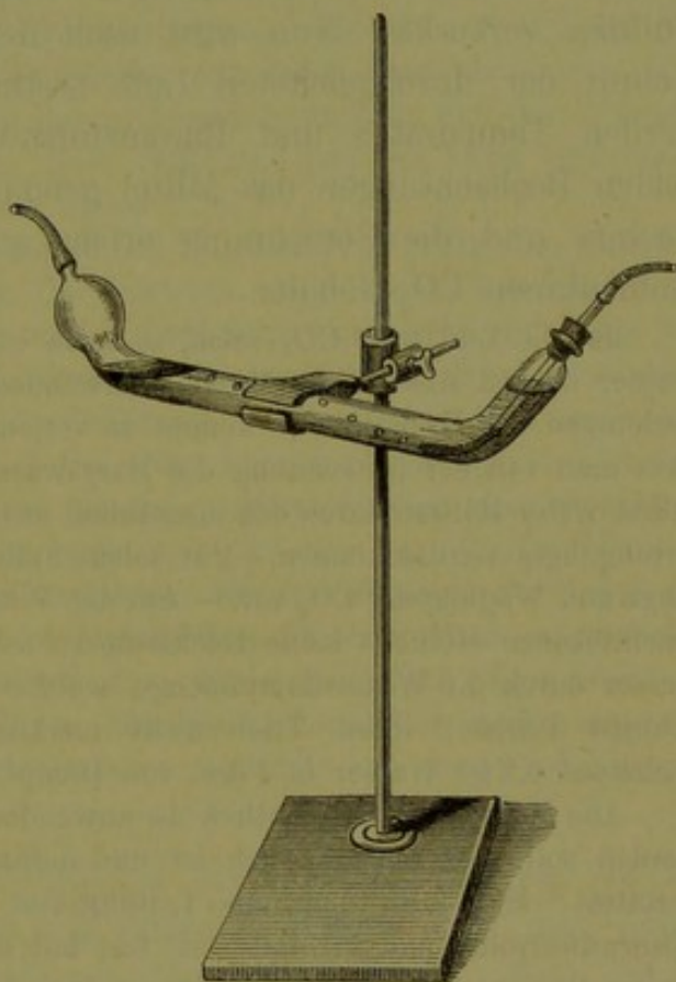
Kohlensäure-Bestimmung.
