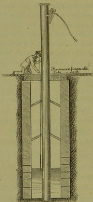
Messung des Grundwasserstandes.
