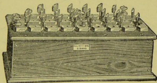
FIG. 14.—RESISTANCE-BOX.
