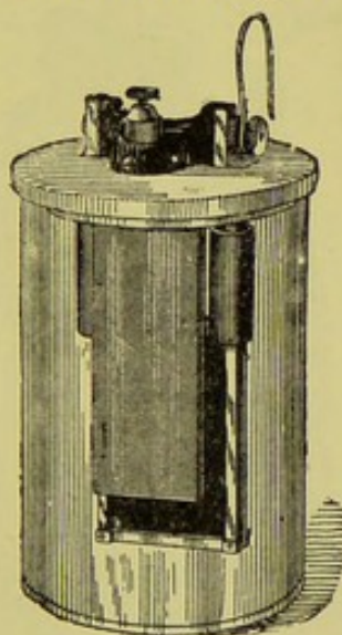
FIG. 7.—EDISON-LALANDE CELL.
