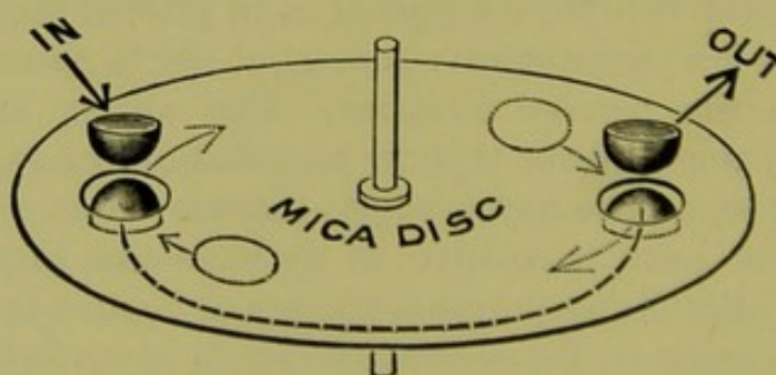
FIG. 113.—REVOLVING DISC RECTIFIER.
