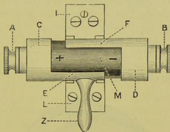
FIG. 26.—COMMUTATOR OF RUHKORFF.
