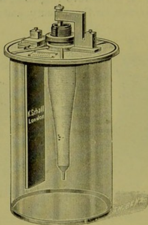
FIG. 105.—WEHNELT INTERRUPTER.
