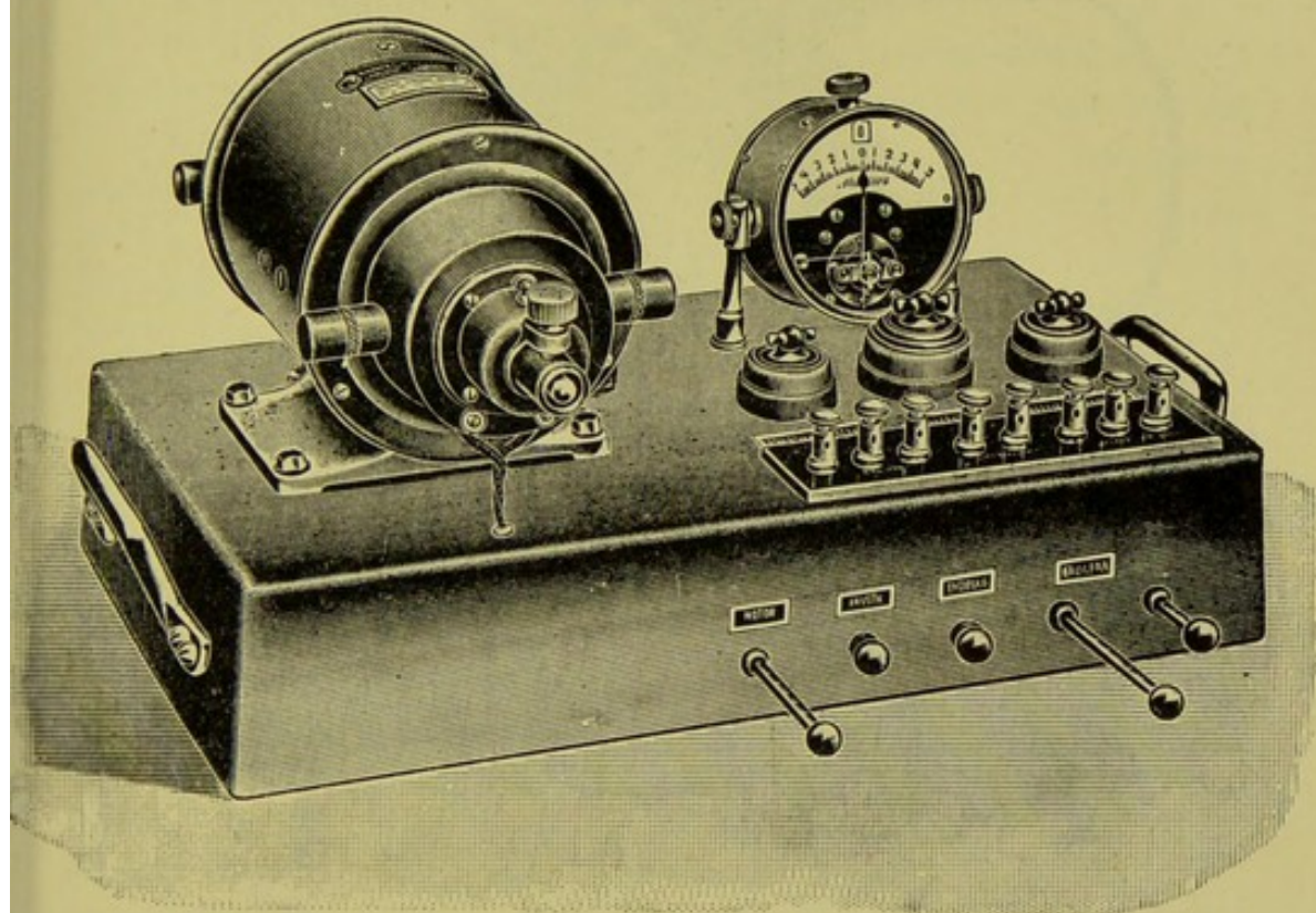
FIG. 86.—PANTOSTAT.
