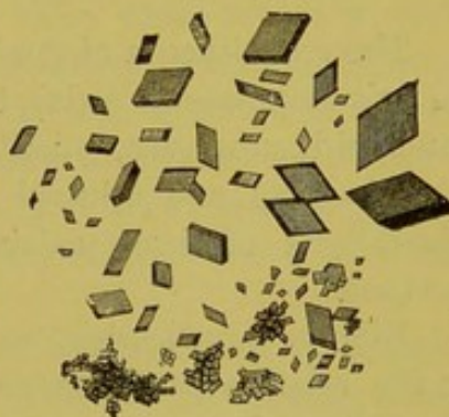
FIG. 24.—Hæmatoidin crystals.
