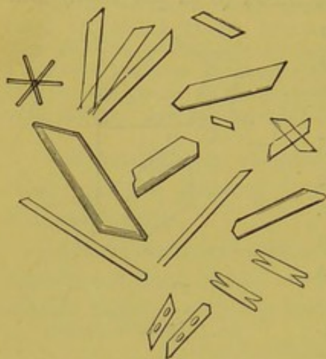
FIG. 2.—Inositol crystals.
