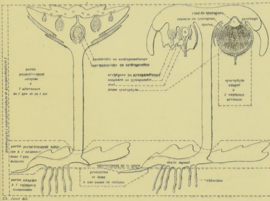
FIG. 2. — Schéma contenant l'orthophyte d'une Hépatique ( Marchantia polymorpha )
