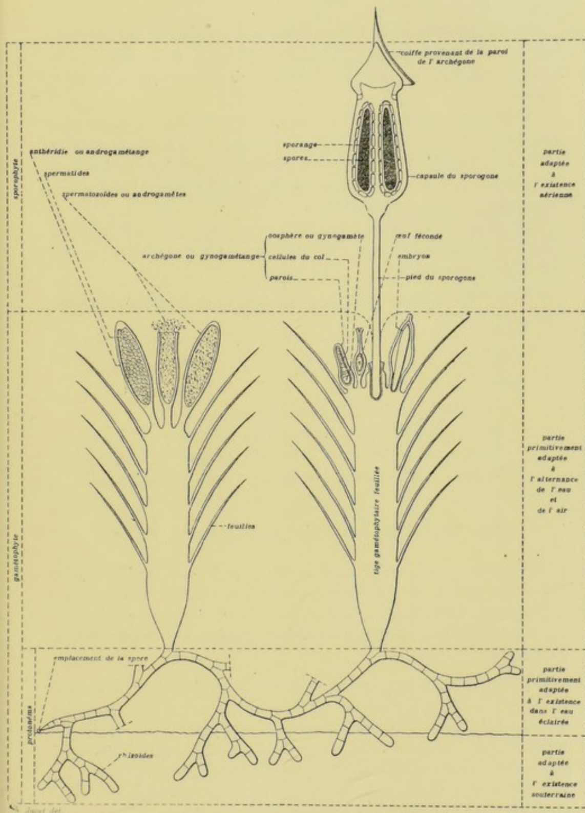
FIG. 1. — Schéma contenant l'orthophyte d'une Mousse ( Atrichum undulatum )
