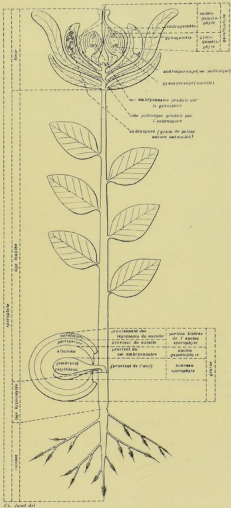
FIG. 5. — Schéma contenant l'orthophyte d'une Phanérogame.
