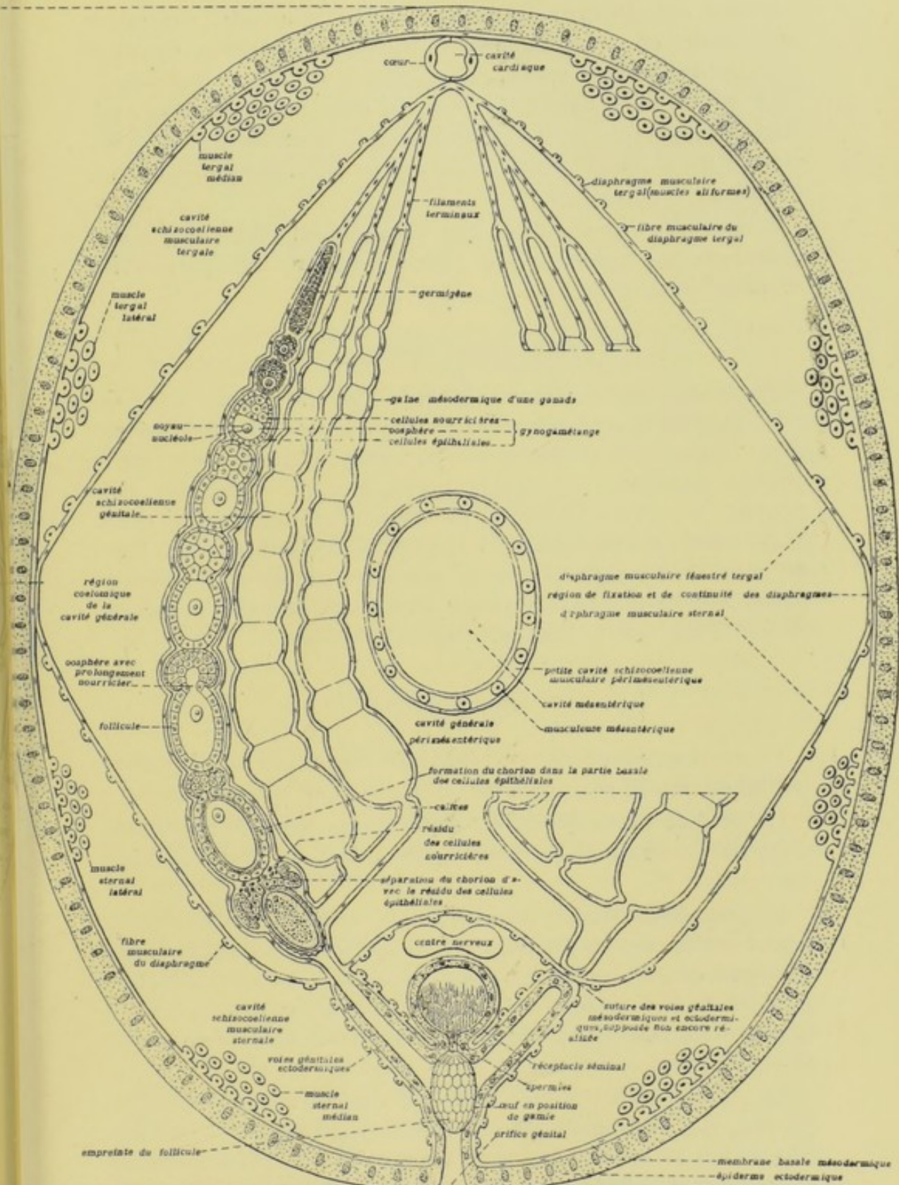
FIG. 7. — Schéma d'une coupe transversale de l'abdomen d'un Insecte montrant la disposition des ovaires et leurs rapports avec les membranes mésodermiques.
