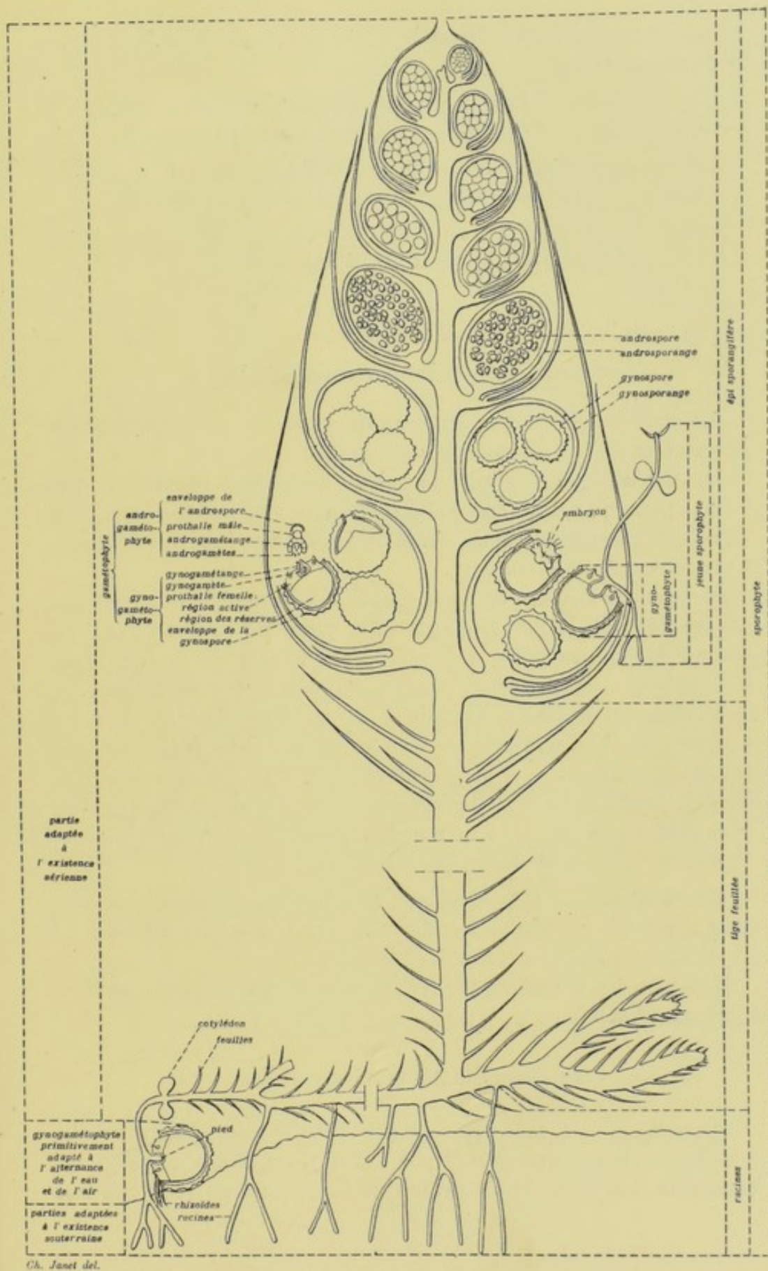
FIG. 3. — Schéma contenant l'orthophyte d'une Lycopodiinée hétérosporee (Selaginella). Il arrive parfois, comme on l'a figuré ici, qu'une jeune plantule se développe sur l'épi.
