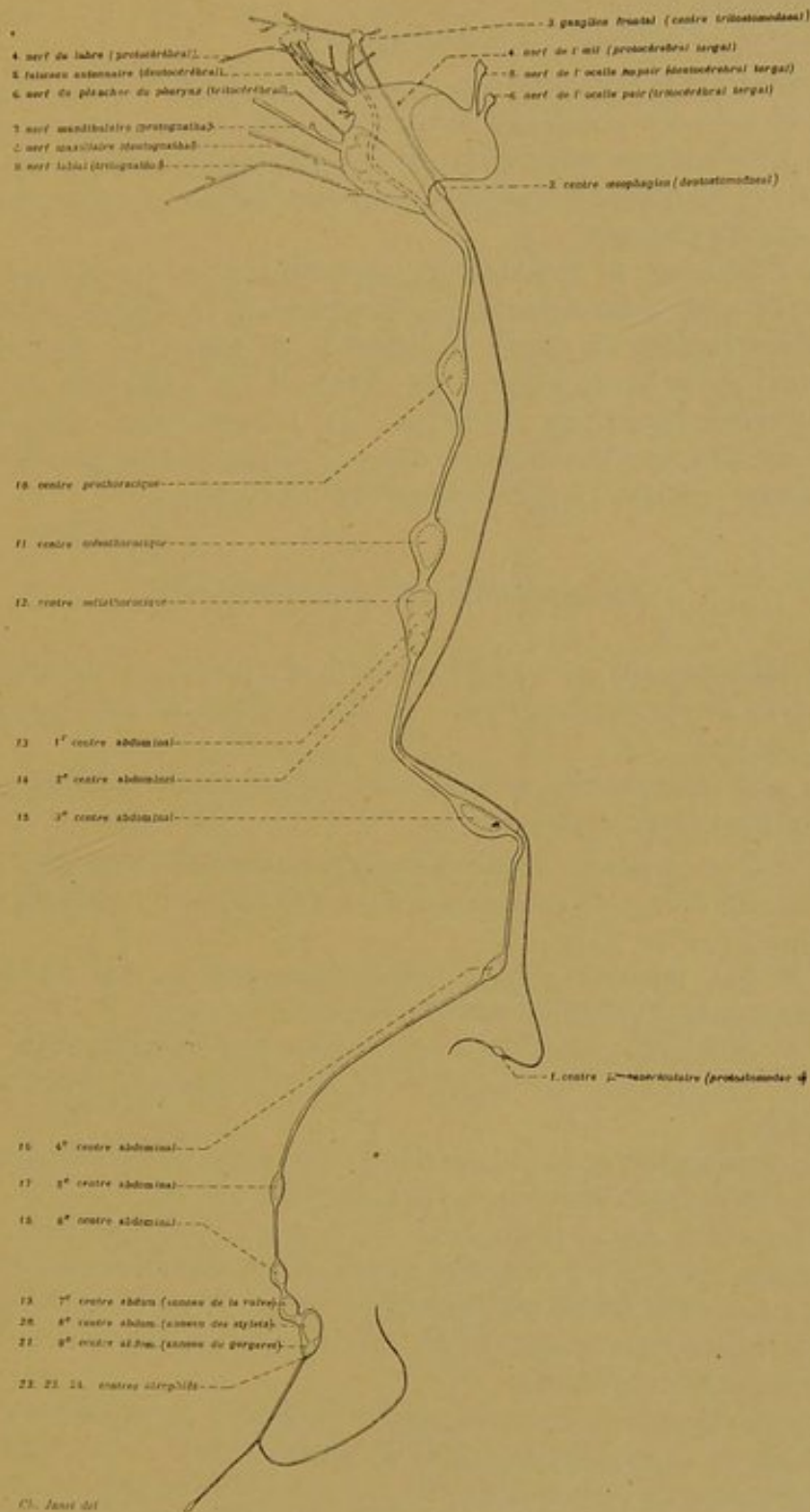
Fig. 2. — Schema morphologique du système nerveux de la Myrmica .
