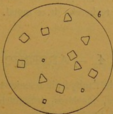
Fig. 6. — Chlorure d'argent.
