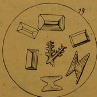
Fig. 19. — Phosphate ammoniaco-magnésien.
