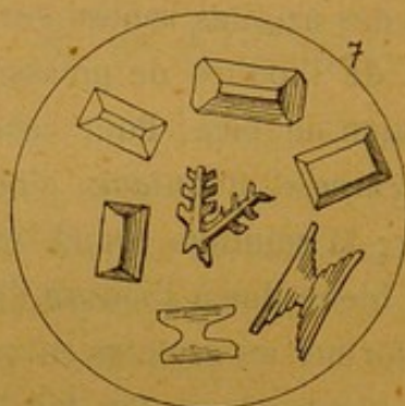
Fig. 7. — Phosphate ammoniaco-magnésien.
