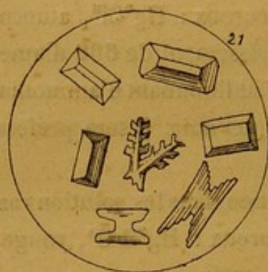
Fig. 21. — Phosphate ammoniaco-magnésien.
