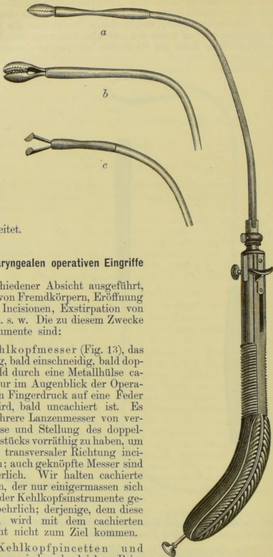
Fig. 14 a u. b. Türk'sche Kehlkopfpincette, a. geschlossen, b. offen. c. Schroetter's Pincette für Trachealtumoren.
